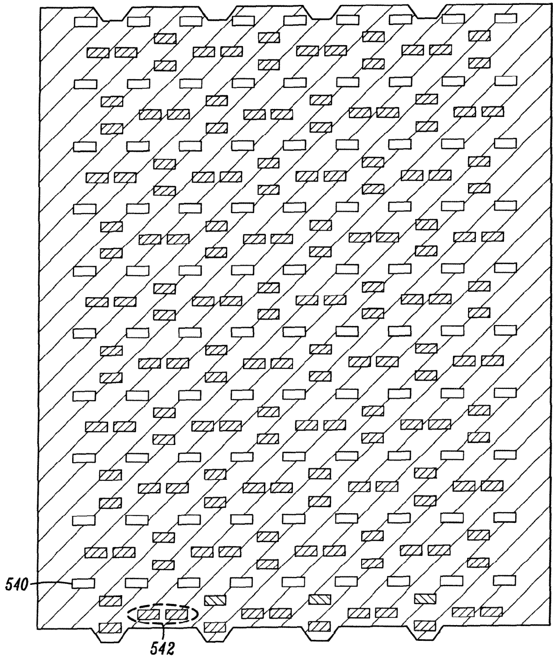
SECTION D-D
