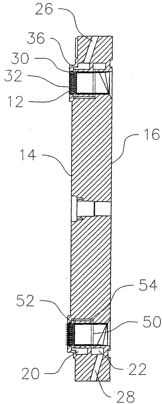
SECTION A-A
