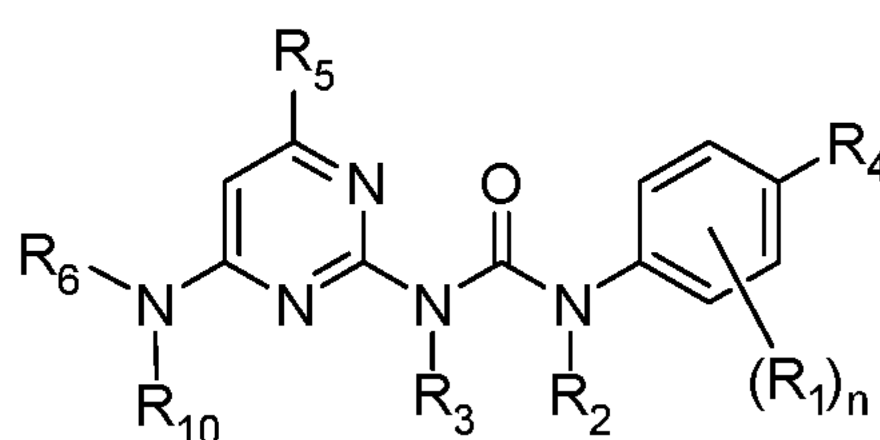
Formula (IIA);
