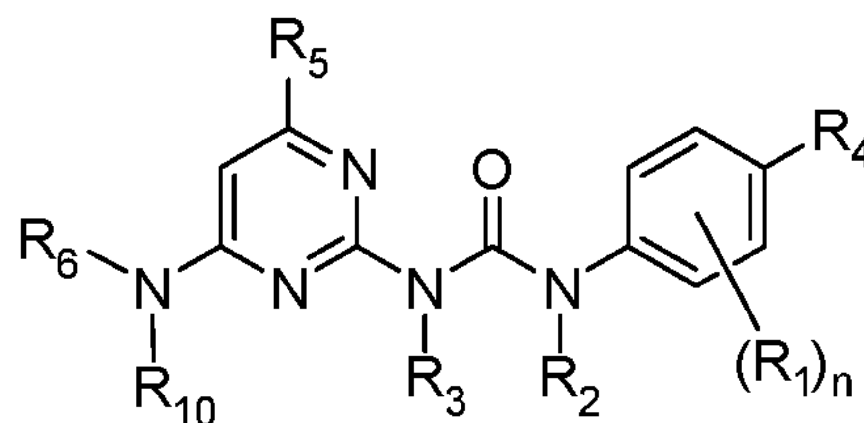
Formula (VI);
