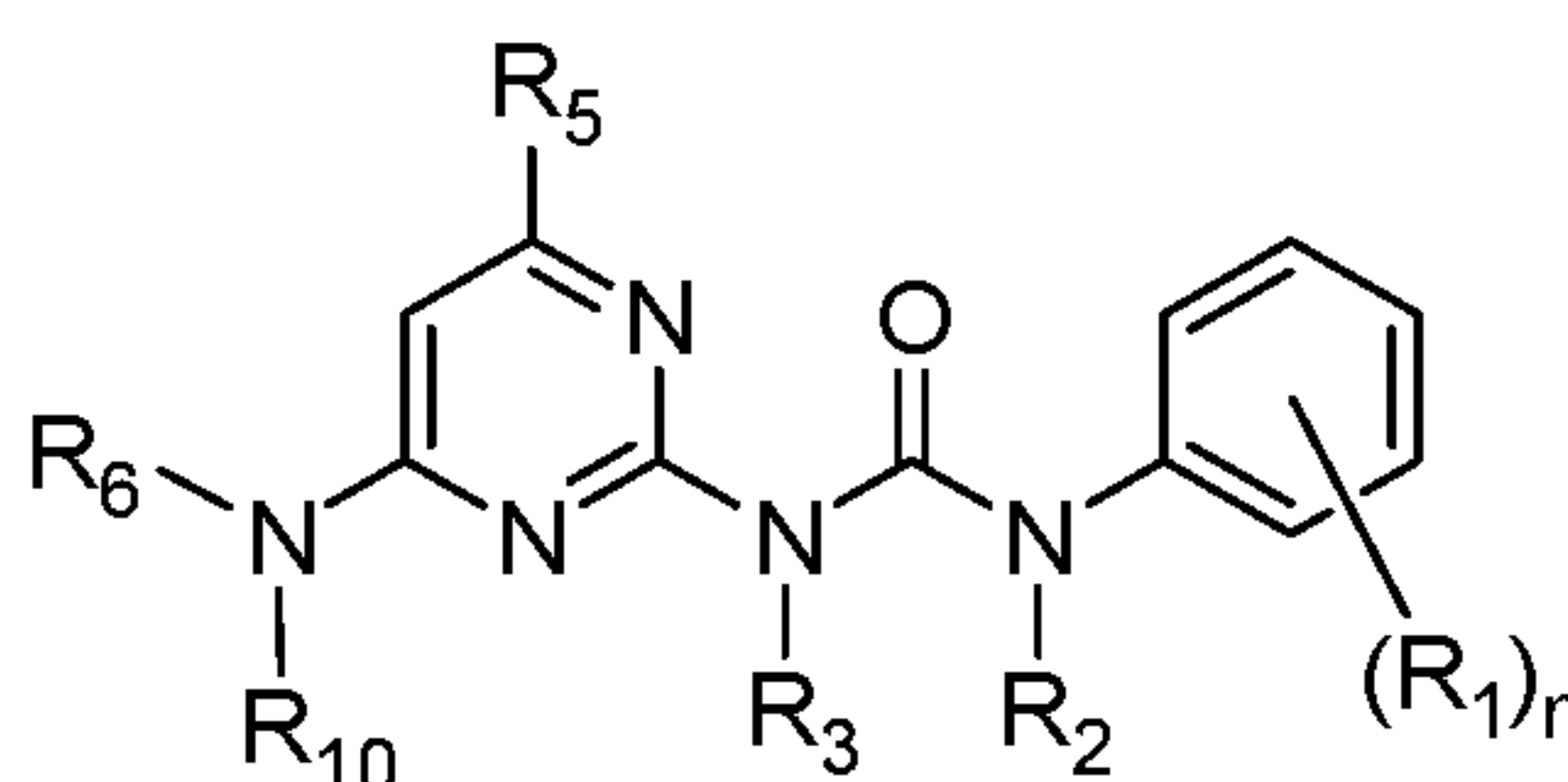
Formula (VI);
