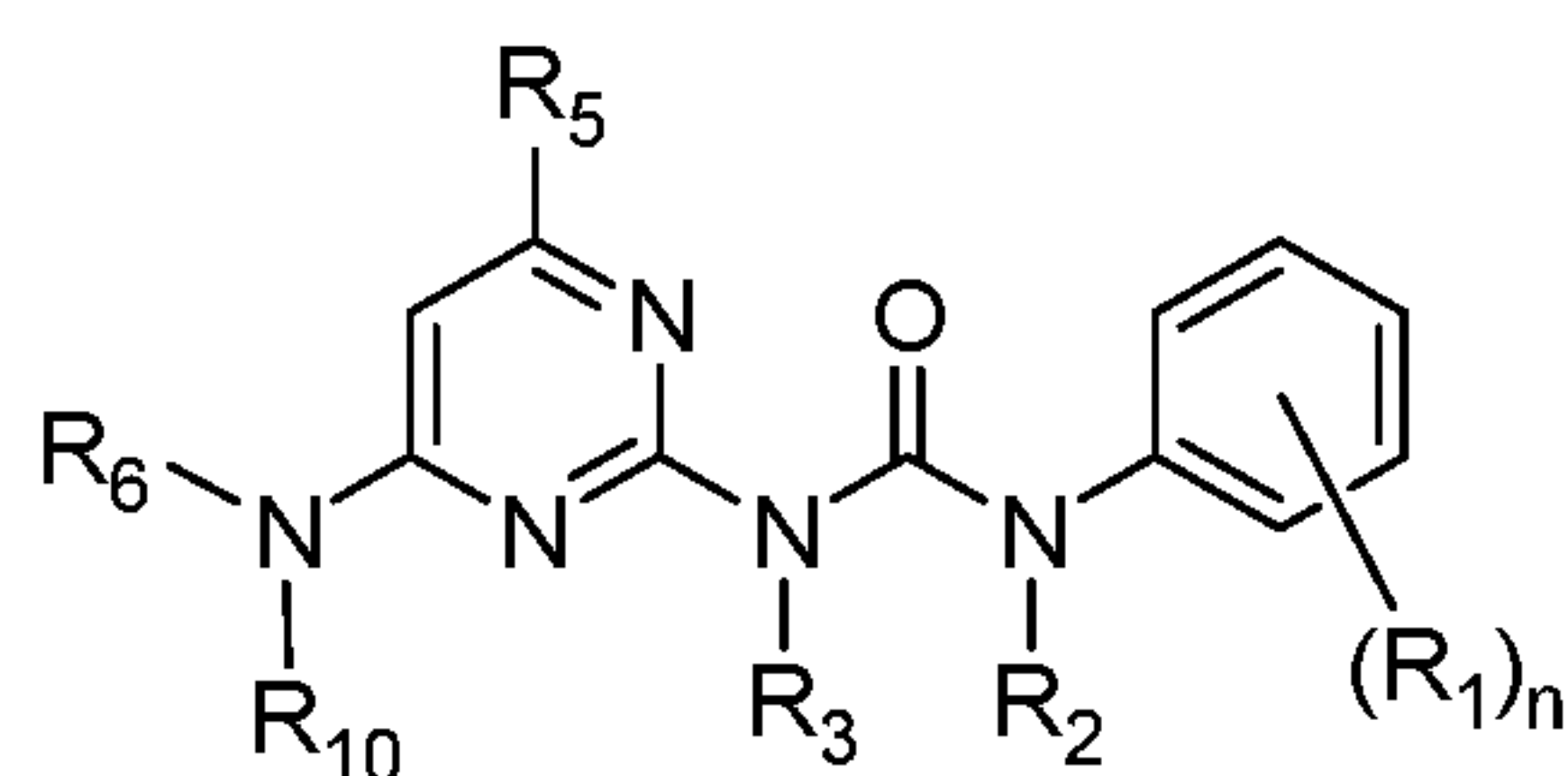
Formula (VI);
