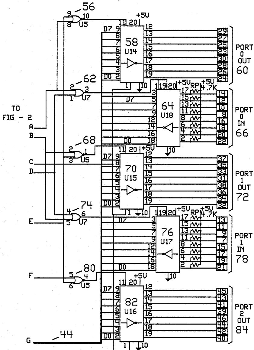
FIG - 2A
