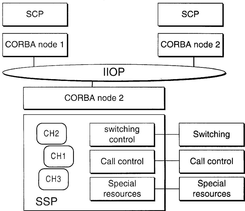
FIG. 5 SSP Server
