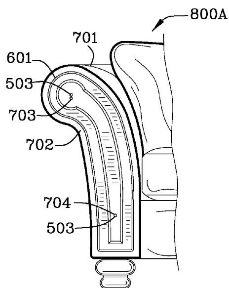
FIG. 8A PRIOR ART
