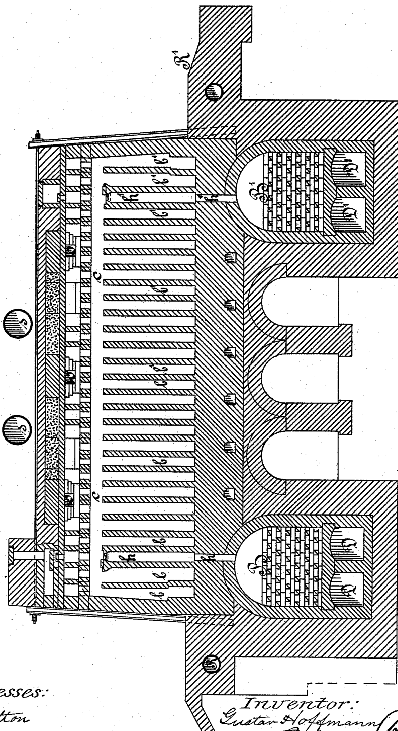
Fig. 2. Section 3-4.
