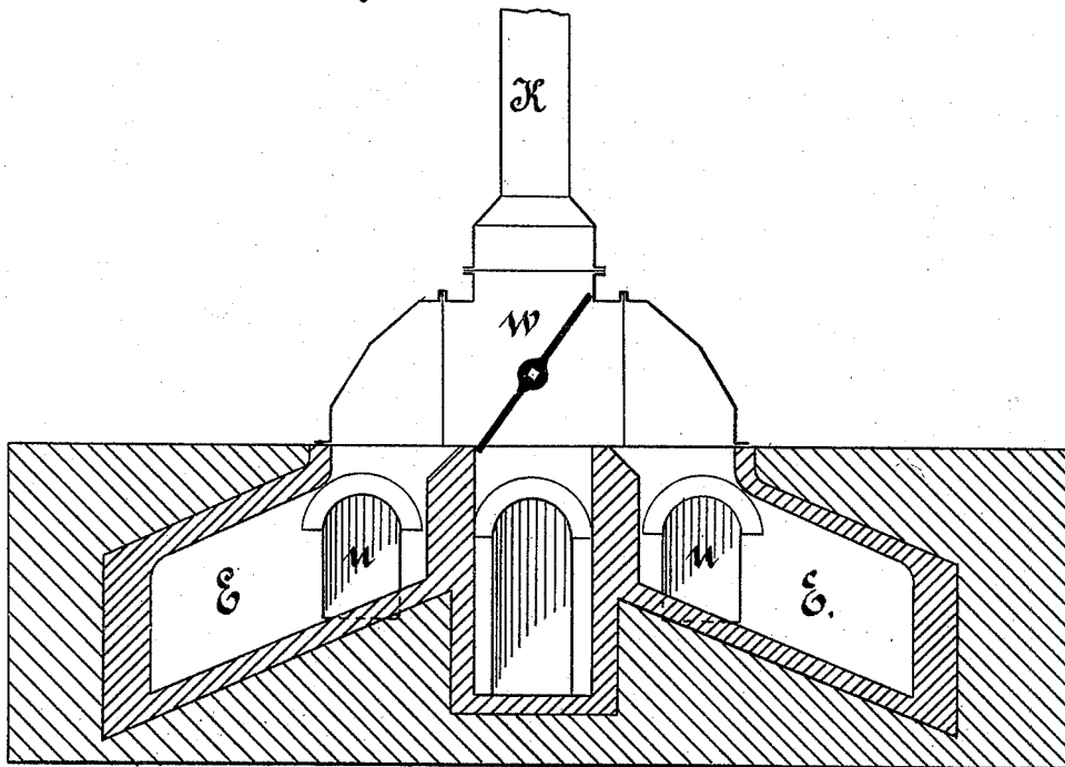
Fig. 6. Section 7-8.
