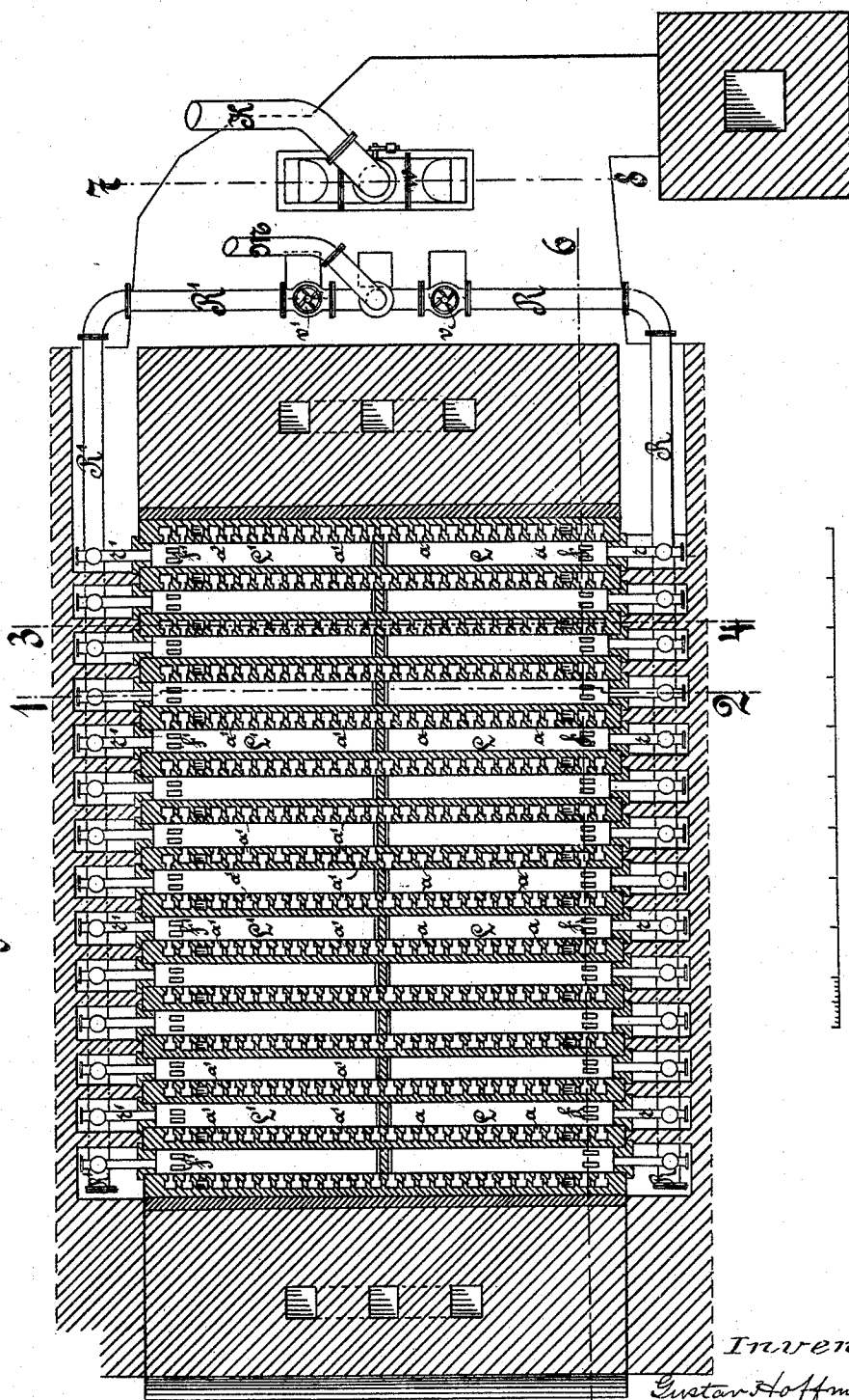
Fig. 4. Section 9-10.
