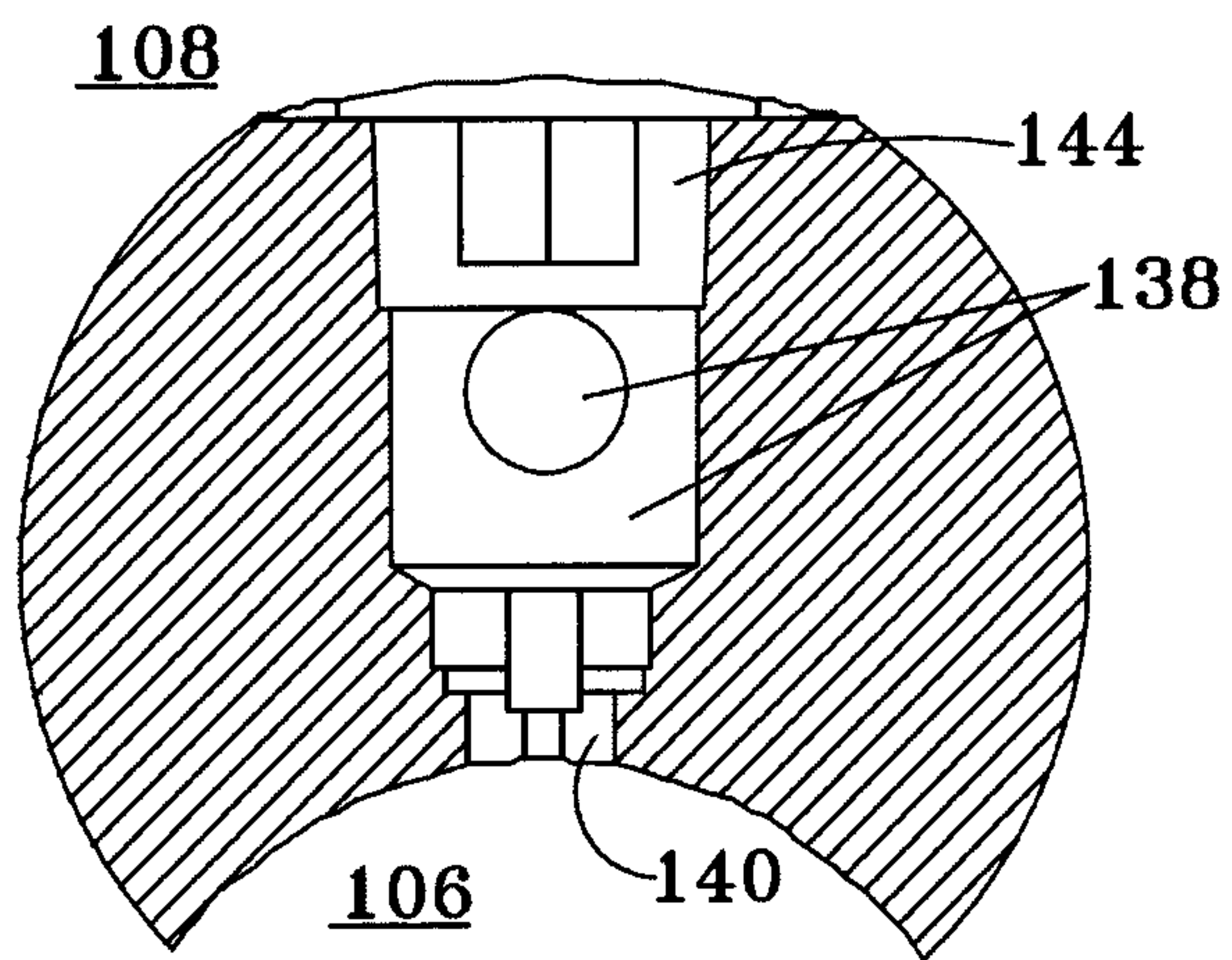
FIG. 9
