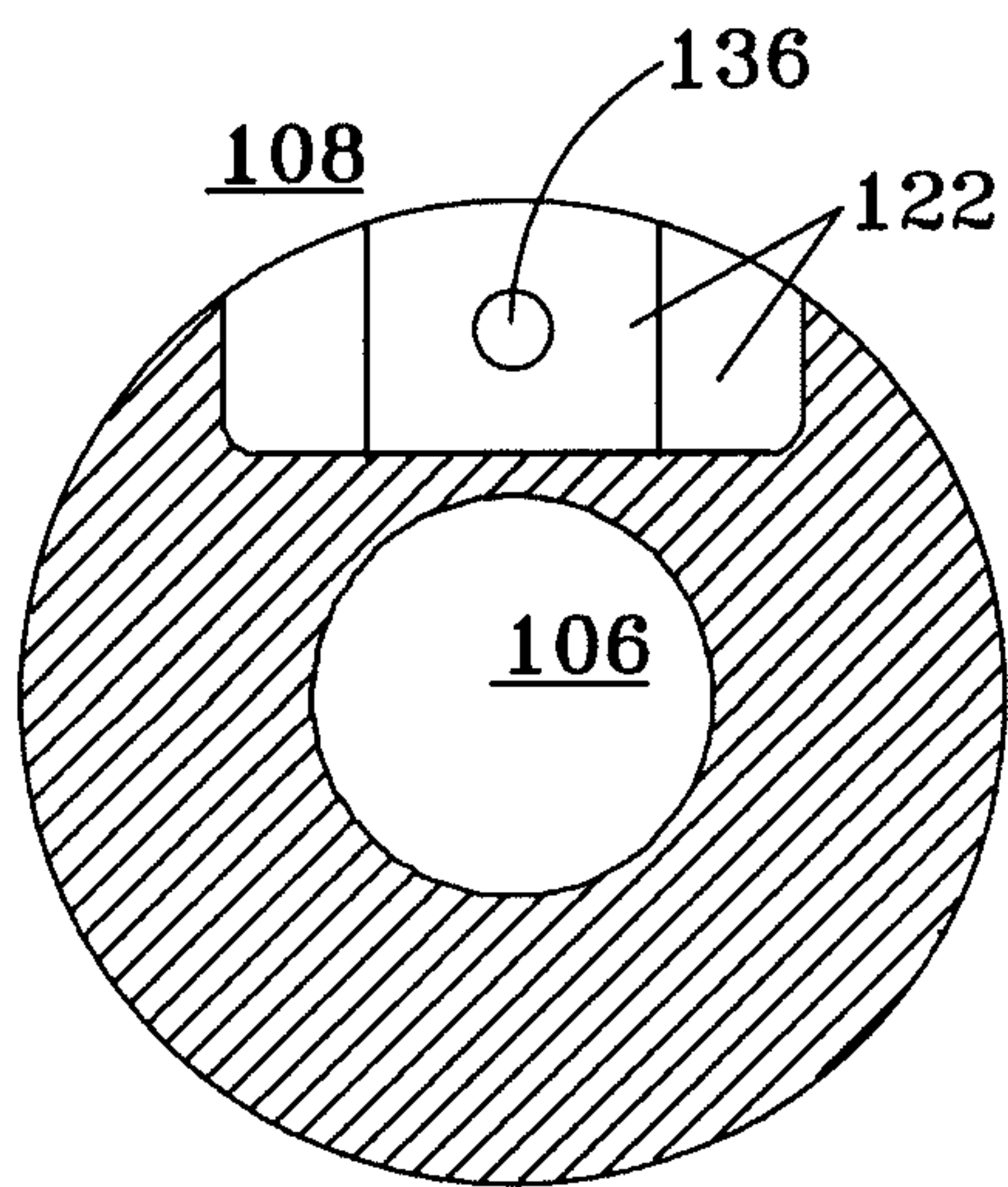
FIG. 10
