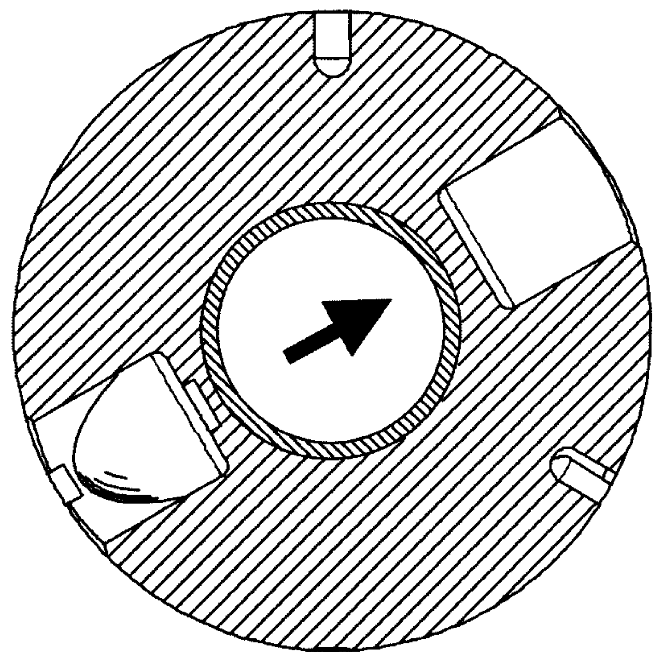
FIG. 23
