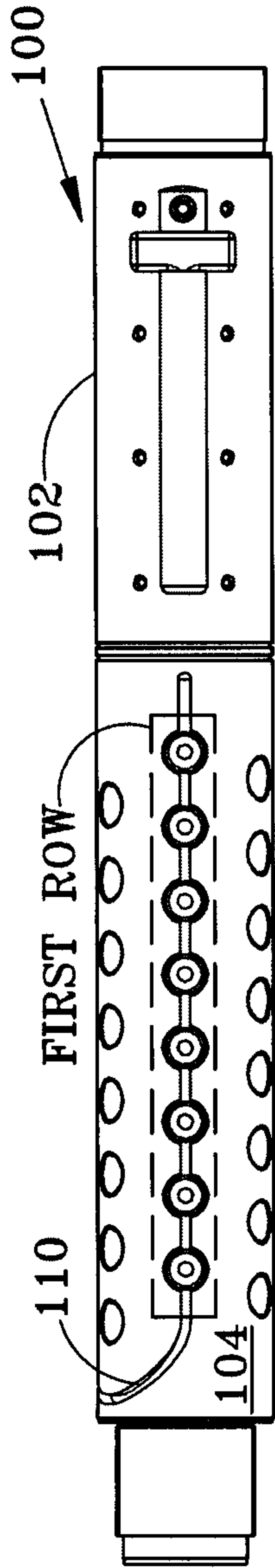
FIG. 14
