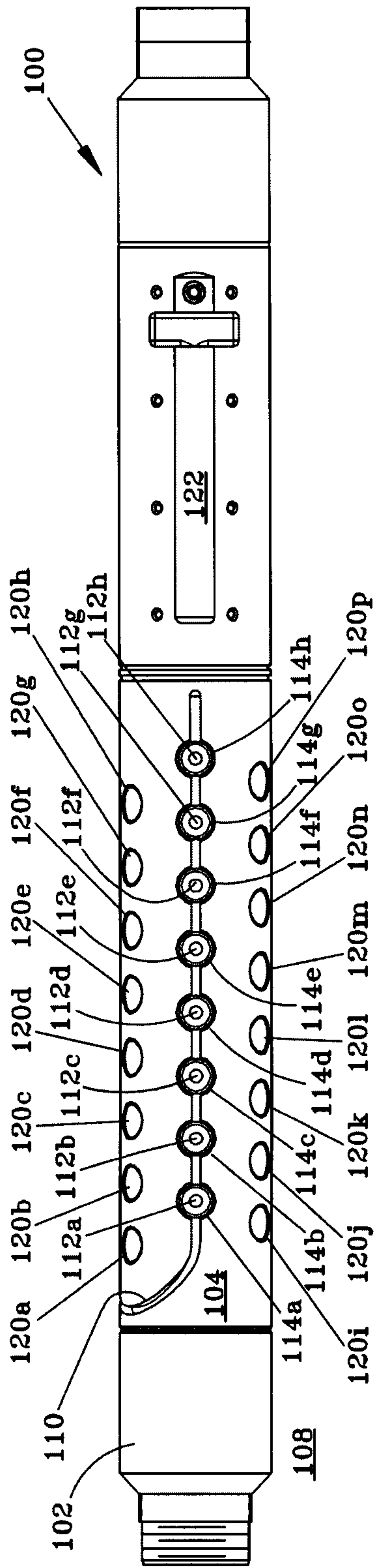
FIG. 1
