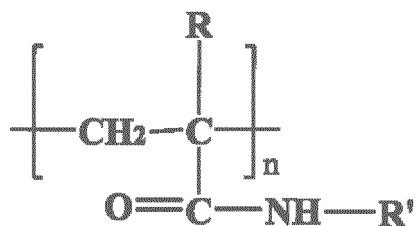
[Chemische Formel 2]
