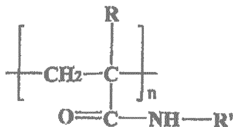
[Formule chimique 2]
