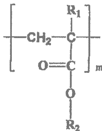
[Formule chimique 2]
