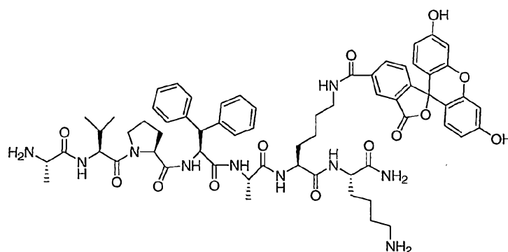
AVP-diPhe-FAM probe
