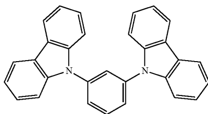
1,3-Bis(N-carbazolyl)benzene
