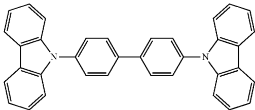
4,4'-Bis(N-carbazolyl)-1,1'-biphenyl
