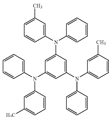
1,3,5-Tris[(3-methylphenyl)phenylamino]benzene
