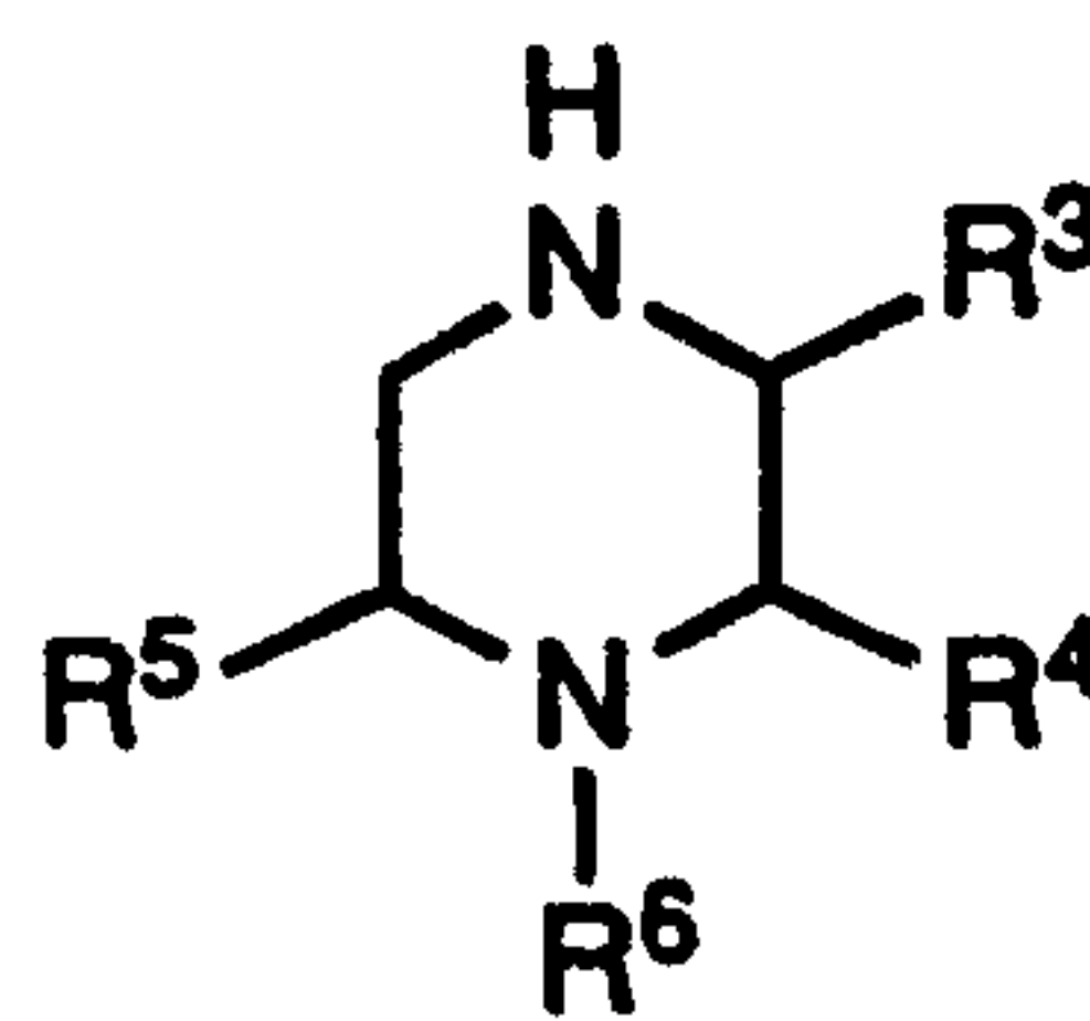
(VII)
