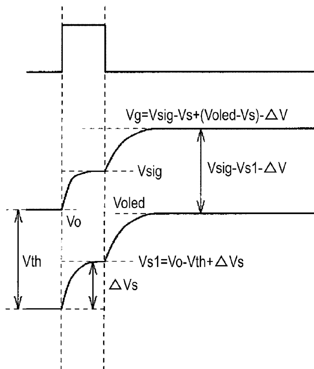
FIG. 12B GATE VOLTAGE V_g
