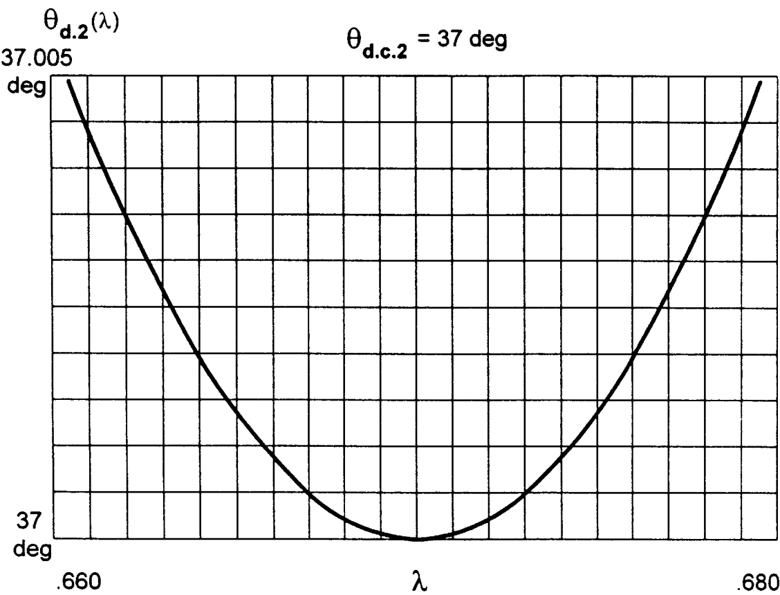
F I G. 27D
