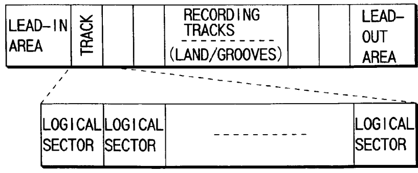
FIG. 2B ←→ 2048 BYTES (2k BYTES)
