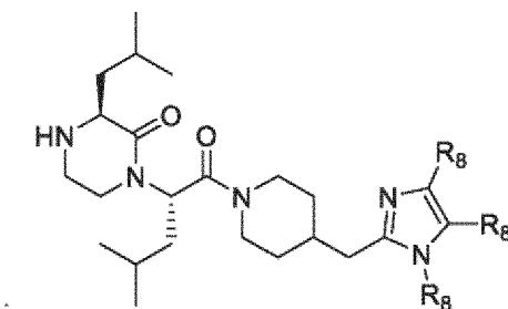
(VIIIf);
