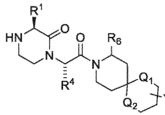
(VIIIg);
