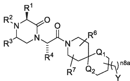
(VIId1);
