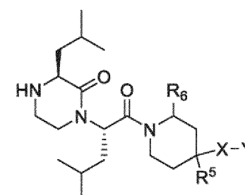
(IVd);
