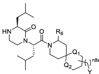
(VIIIk1); or
