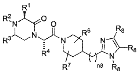
(VIIa);
