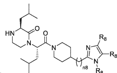
(VIId);
