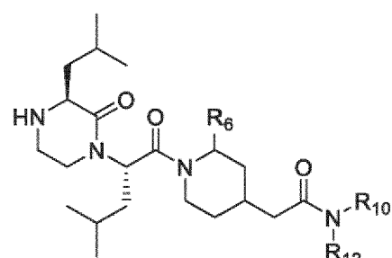
(Vd);
