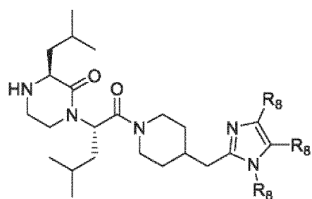
(VIIe);
