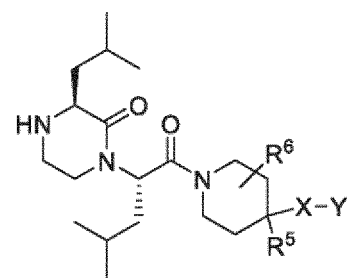
(IIId);
