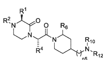
(VIa);
