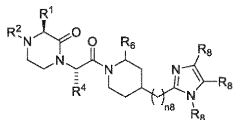
(VIIb);
