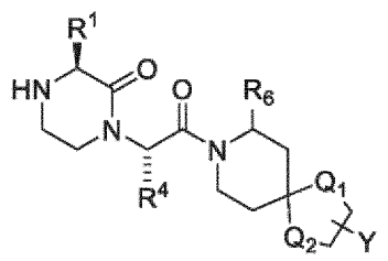
(VIIIg);
