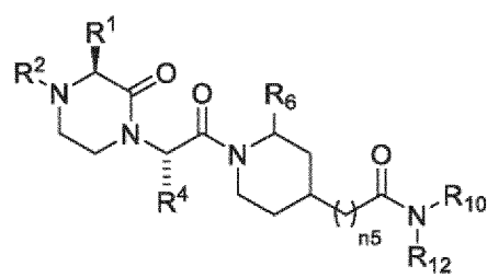
(Va);
