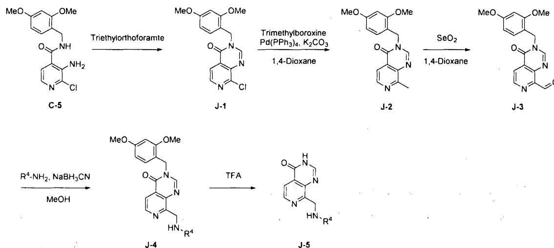
Scheme 10 (Method J)
