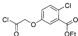
ethyl 2-chloro-5-(2-chloro-2-oxoethoxy)benzoate
