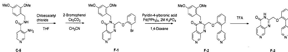
Scheme 6 (Method F)
