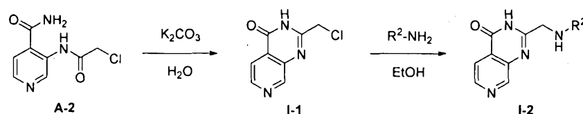
Scheme 9. (Method I)
