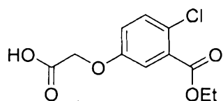
2-(4-chloro-3-(ethoxycarbonyl)phenoxy)acetic acid
