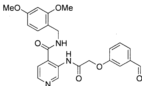
N-(2,4-dimethoxybenzyl)-3-(2-(3-formylphenoxy)acetamido)isonicotinamide
