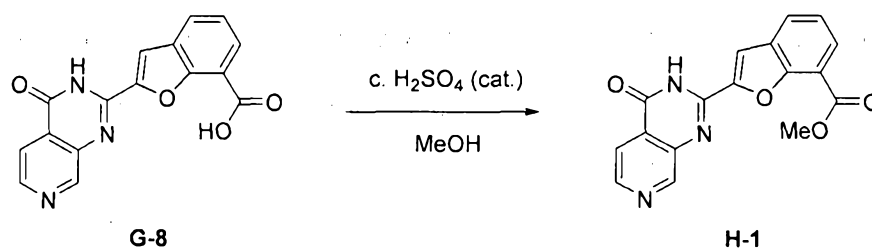
Scheme 8 (Method H)
