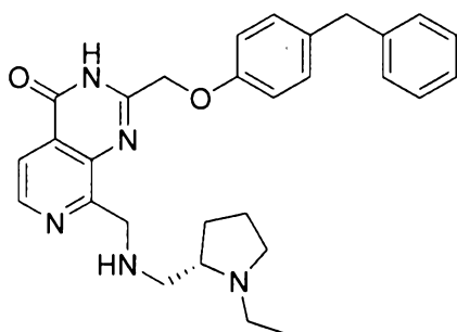
(S)-2-((4-benzylphenoxy)methyl)-8-((((1-ethylpyrrolidin-2-yl)methyl)amino)methyl)pyrido[3,4-d]pyrimidin-4(3H)-one
