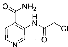
3-(2-chloroacetamido)isonicotinamide
