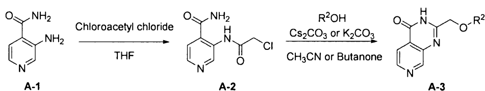
Scheme 1 (Method A)
