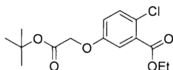
ethyl 5-(2-(tert-butoxy)-2-oxoethoxy)-2-chlorobenzoate
