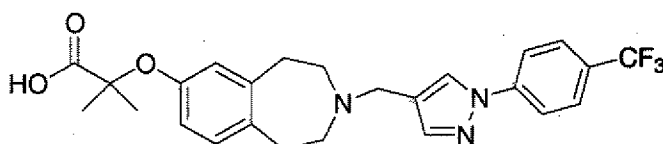
Cmpd 21
