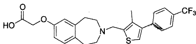
Cpd 15
