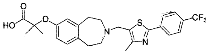
Cpd 6
