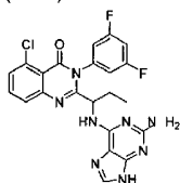
(171)
