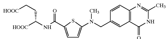
Tomudex
