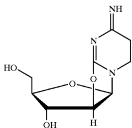
Ancitabine
