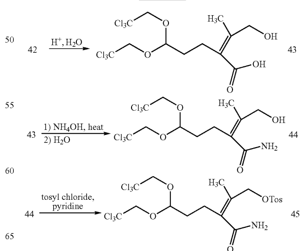
Scheme 12B
