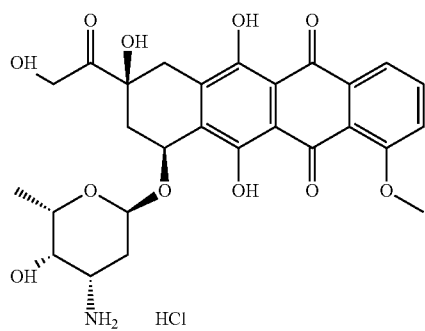
Doxorubicin
