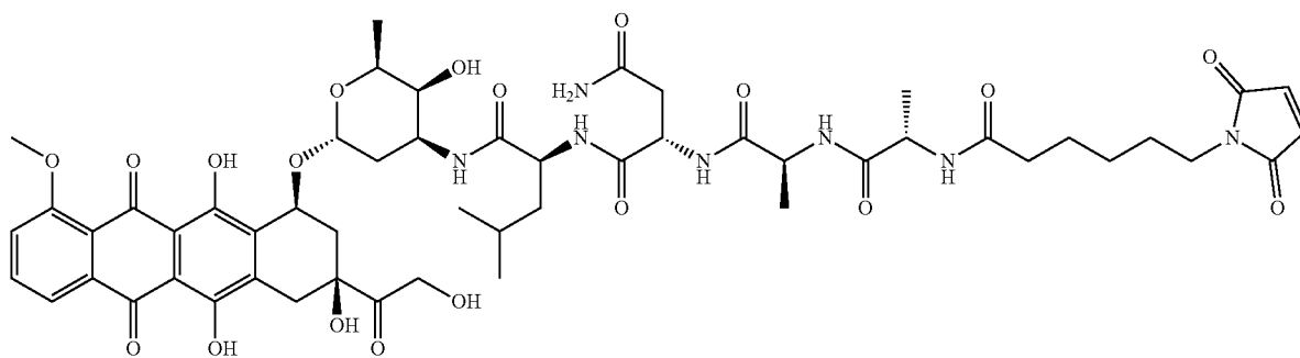
EMC-AANL-Doxorubicin
