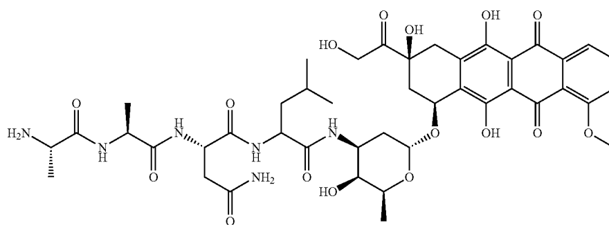
AANL-DOX
