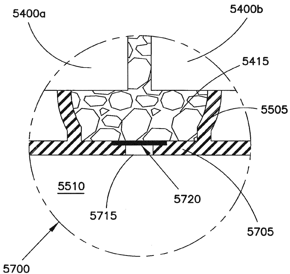
FIG. 57B
