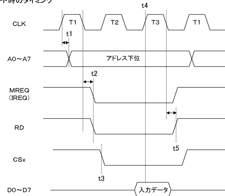
(A) リード時のタイミング
