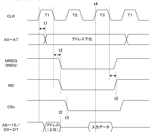
(A) リード時のタイミング
