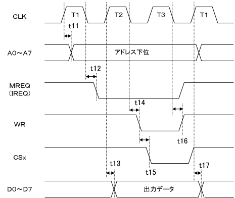
(B) ライト時のタイミング
