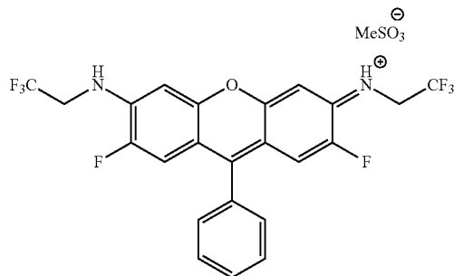
(Z)-N-(2,7-difluoro-9-phenyl-6-((2,2,2-trifluoroethyl)amino)-3H-xanthen-3-ylidene)-2,2,2-trifluoroethan-1-aminium methanesulfonate
