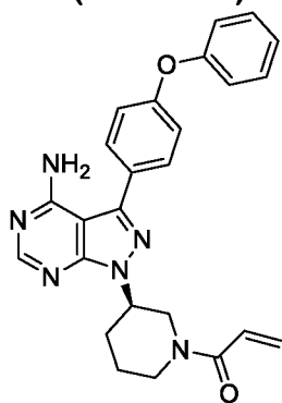
PCI-32765 (Ibrutinib)
