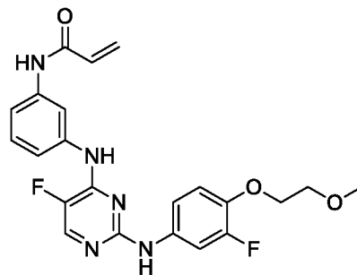
AVL-292
