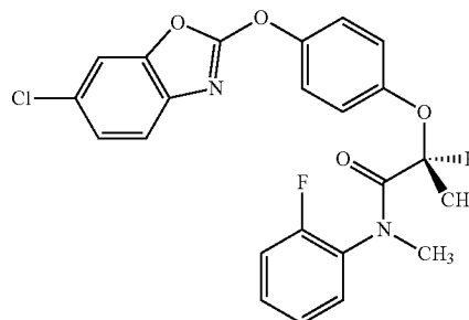
(2S)-2-{4-[(6-chloro-1,3-benzoxazol-2-yl)oxy]phenoxy}-N-(2-fluorophenyl)-N-methylpropanamide
