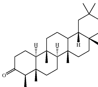
Friedelin
