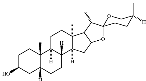
Sarsasapogenin
