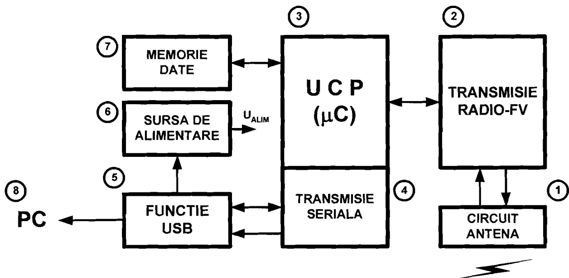
Fig.5 Schema bloc detaliată a cuplului activ pentru controlul traficului de rețea
