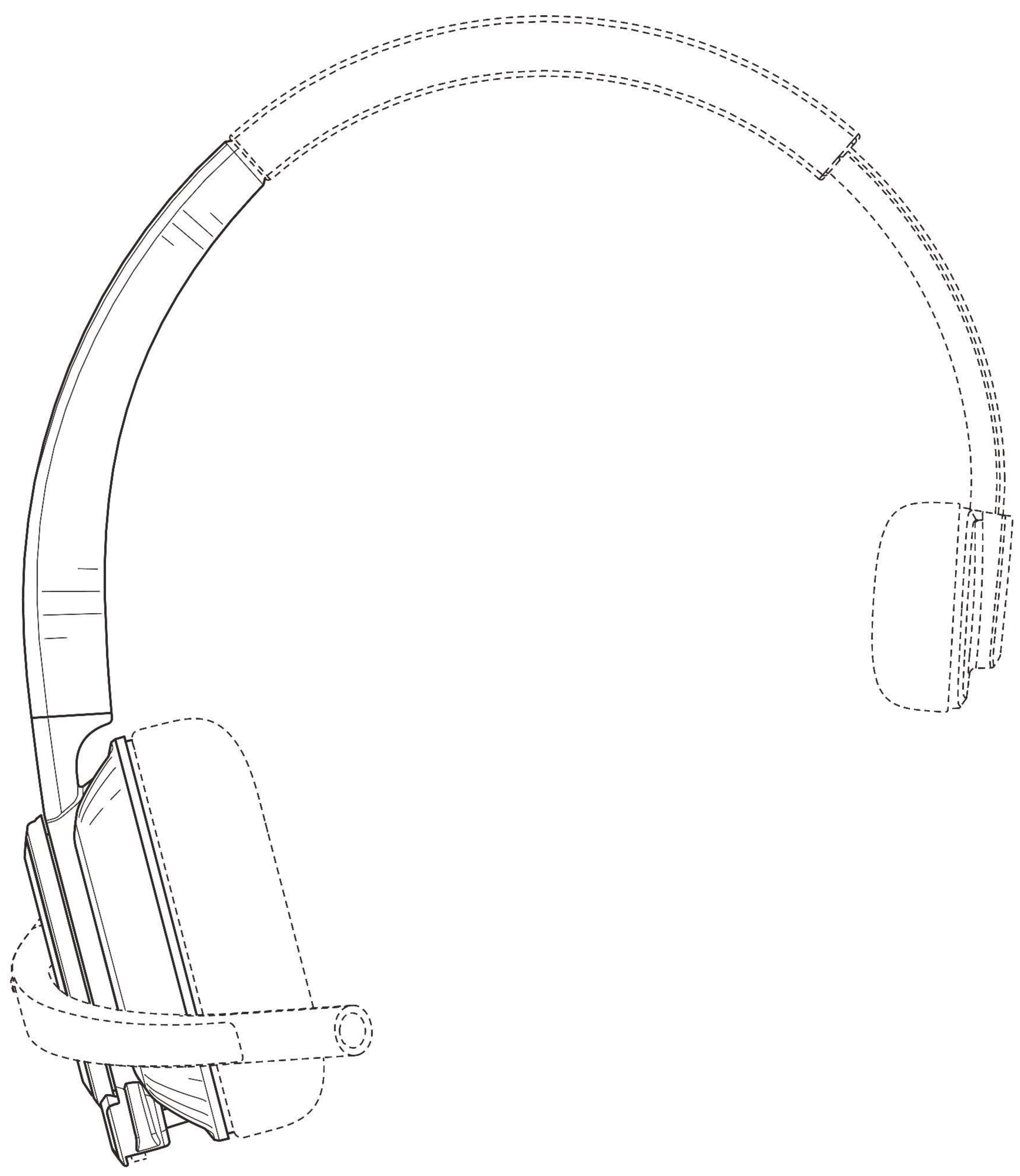
【前視圖】
