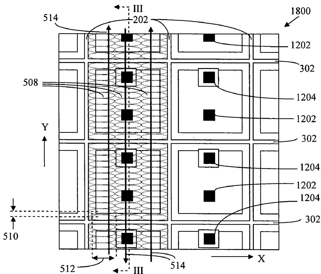
FIG. 21A
