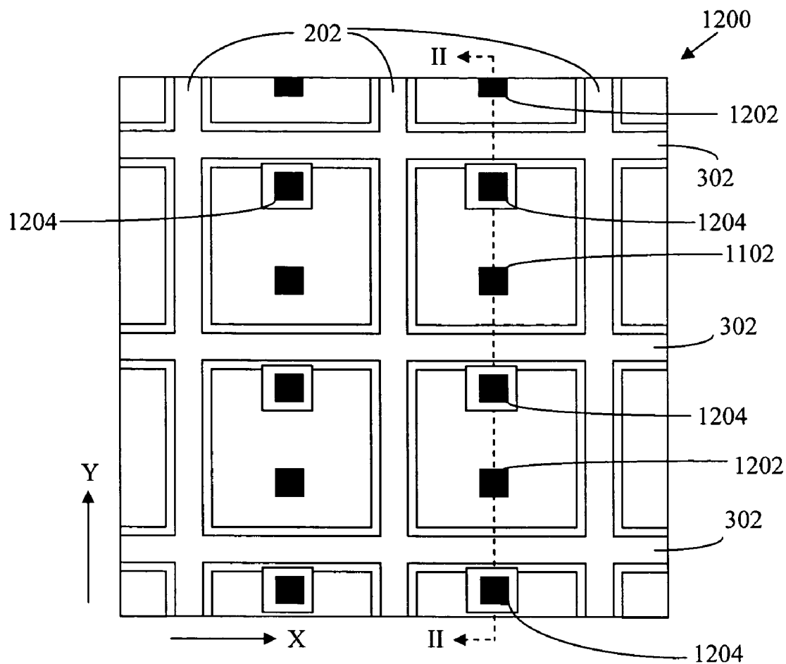
FIG. 14A
