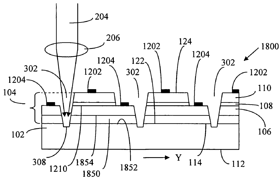
FIG. 20B
