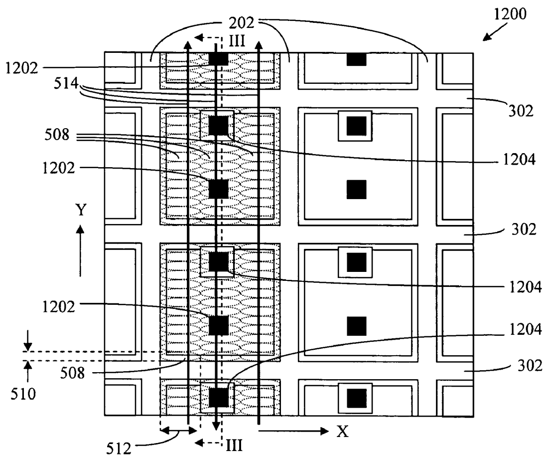
FIG. 15A
