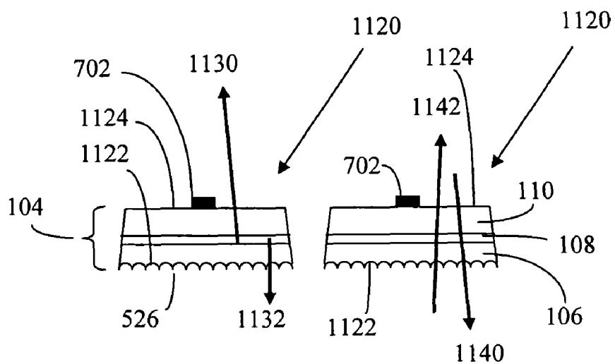
FIG. 11A
