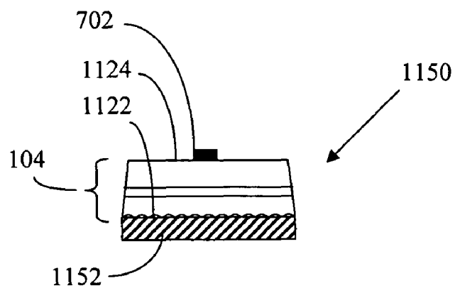
FIG. 11B
