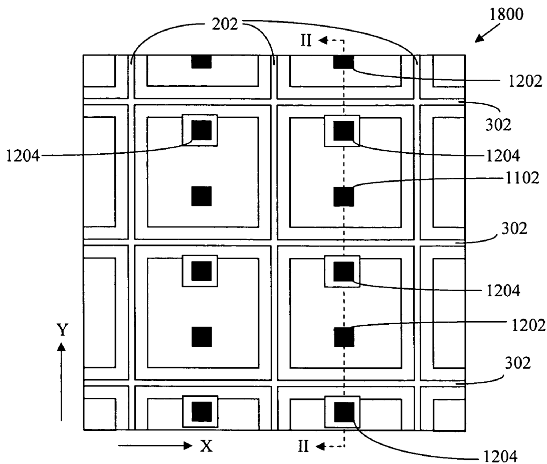
FIG. 20A
