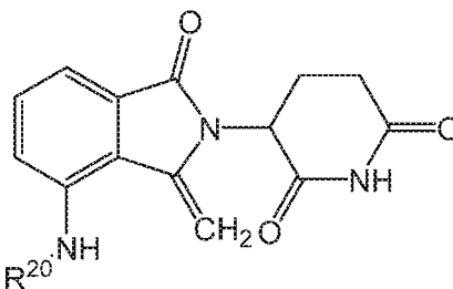
(XVIII)
