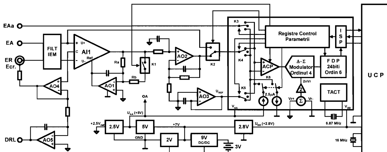
Fig.5 Schema electronică generală a unui circuit pentru măsurarea impedenței de contact între piele și electrodul activ de măsurare neinvazivă a biosemnalelor, conform invenției
