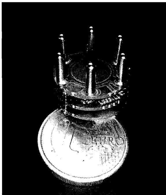
Fig.6 Fotografia unui nod de măsurare biosemnale, prevăzut cu circuit pentru măsurarea impedenței de contact între piele și electrodul activ de măsurare neinvazivă a biosemnalelor, realizat conform invenției
