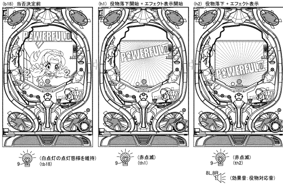
(b18)~(g1)における役物動作の詳細説明図
