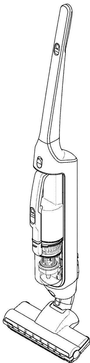
【立體圖1】
