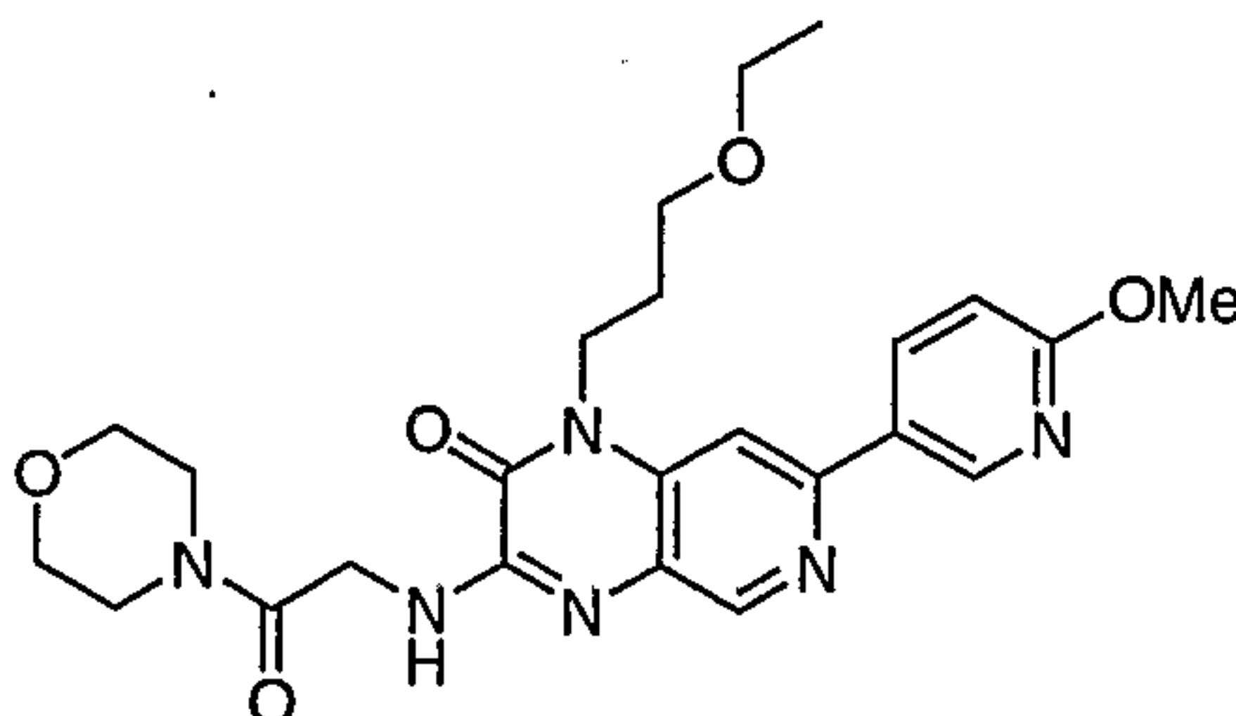
3-(2-morpholino-2-oxoethylamino)-1-(3-ethoxypropyl)-7-(6-methoxypyridin-3-yl)pyrido[3,4-b]pyrazin-2(1H)-one
