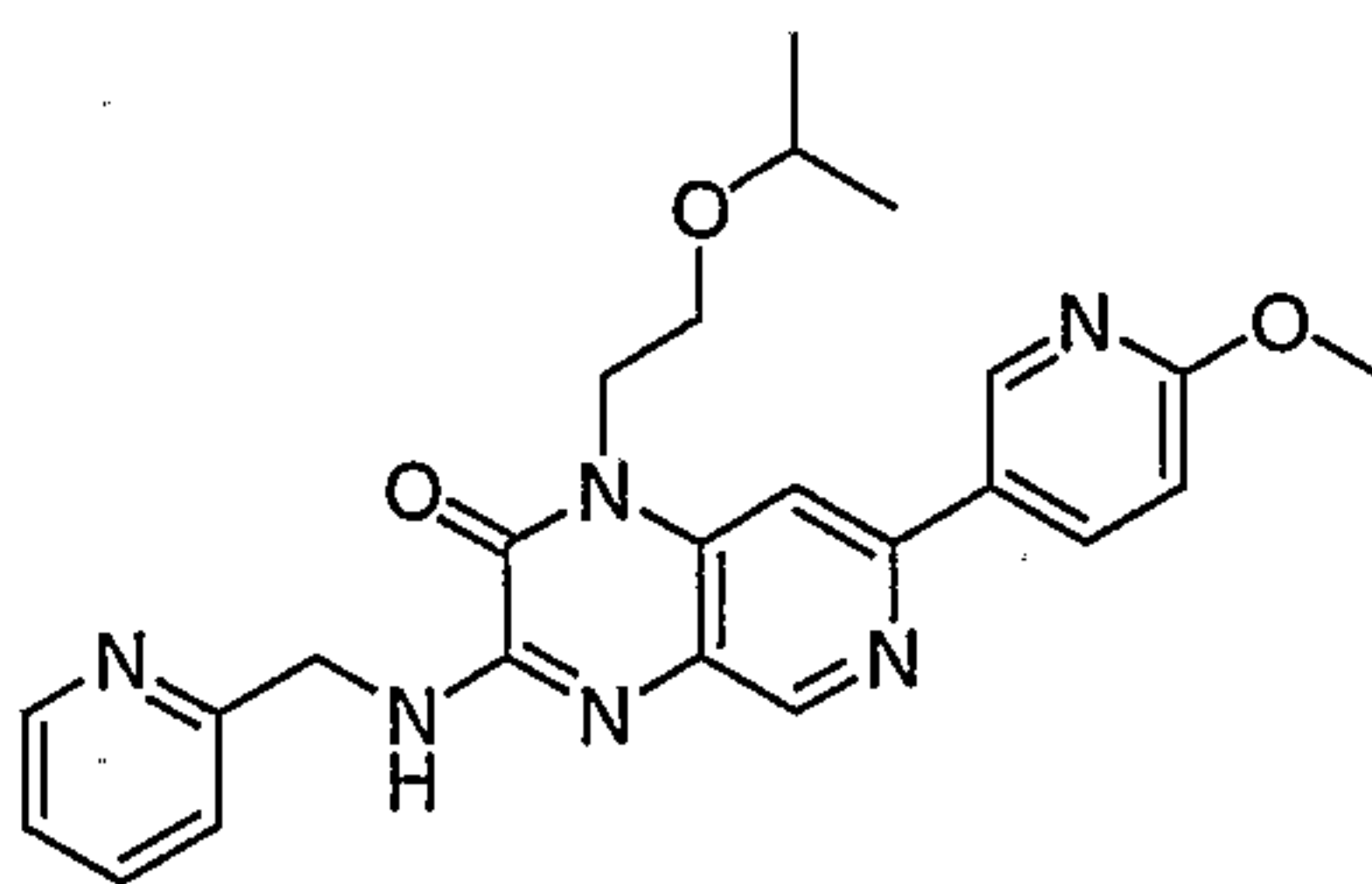
3-((pyridin-2-yl)methylamino)-1-(2-isopropoxyethyl)-7-(6-methoxypyridin-3-yl)pyrido[3,4-b]pyrazin-2(1H)-one
