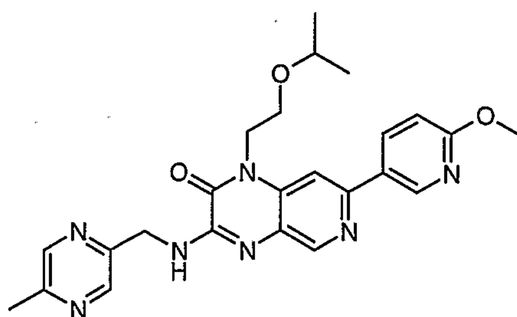
1-(2-isopropoxyethyl)-7-(6-methoxypyridin-3-yl)-3-[[5-methylpyrazin-2-yl)methyl]amino]pyrido[3,4-b]pyrazin-2(1H)-one.
