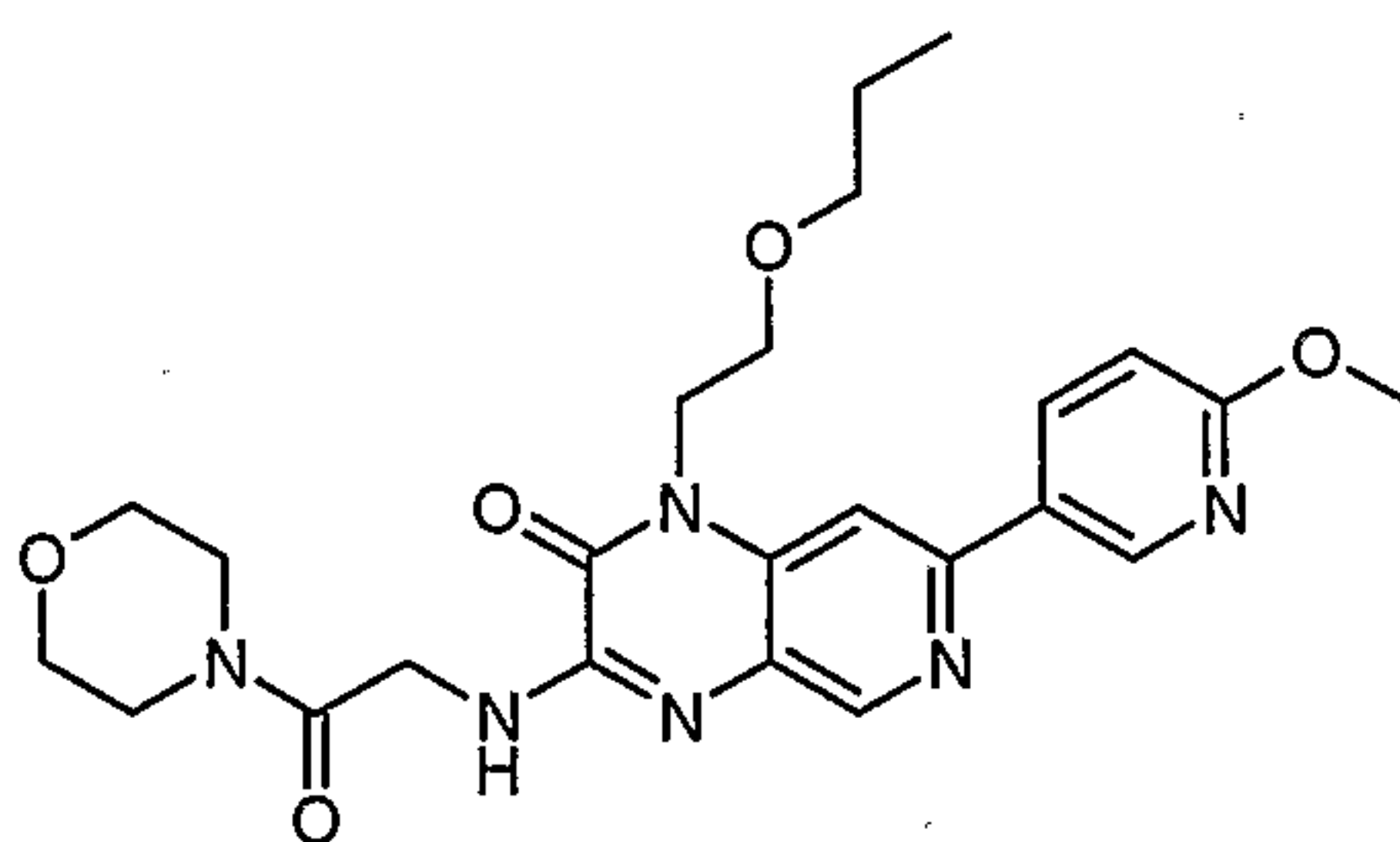
3-(2-morpholino-2-oxoethylamino)-7-(6-methoxypyridin-3-yl)-1-(2-propoxyethyl)pyrido[3,4-b]pyrazin-2(1H)-one
