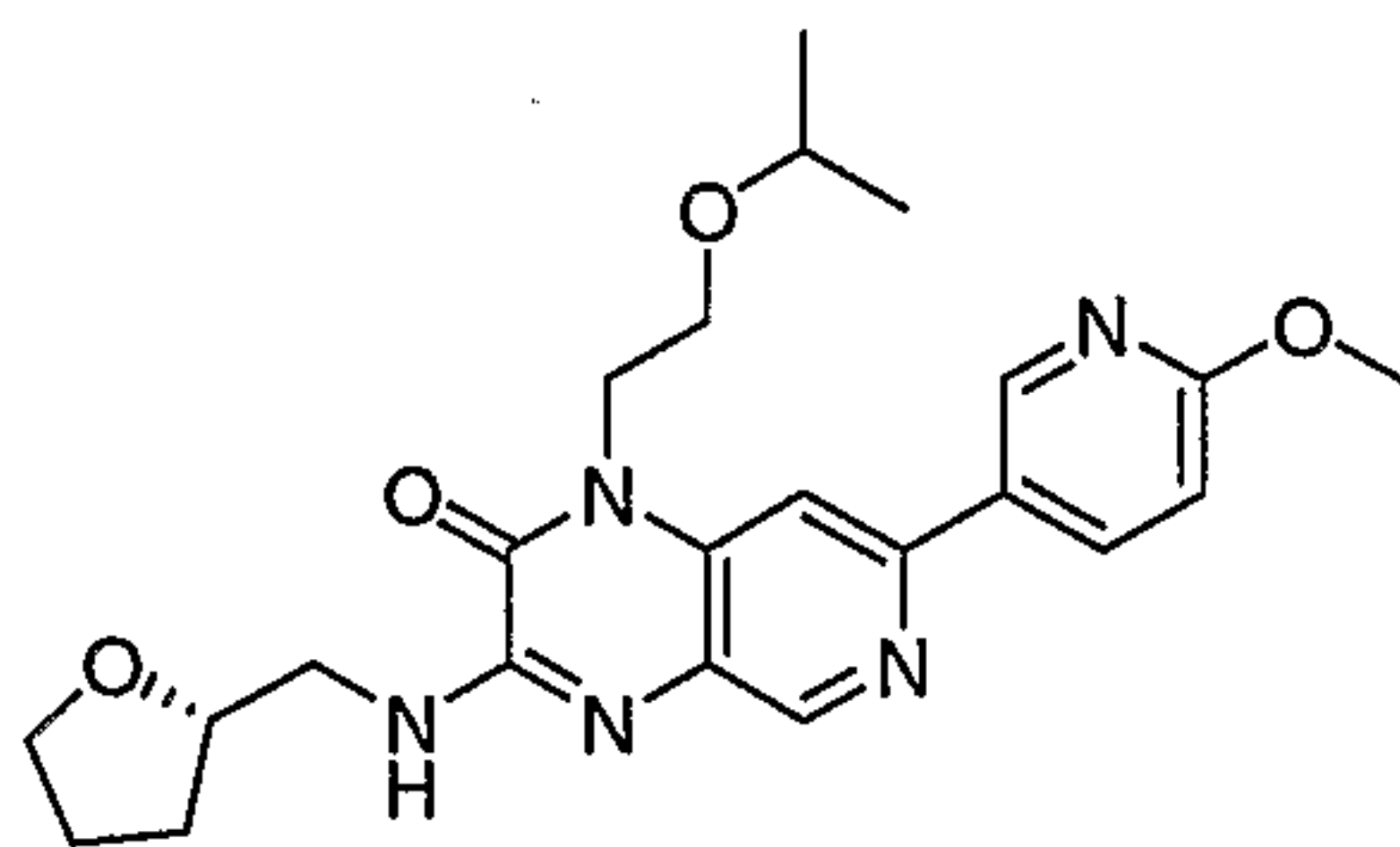
3-(((S)-tetrahydrofuran-2-yl)methylamino)-1-(2-isopropoxyethyl)-7-(6-methoxypyridin-3-yl)pyrido[3,4-b]pyrazin-2(1H)-one
