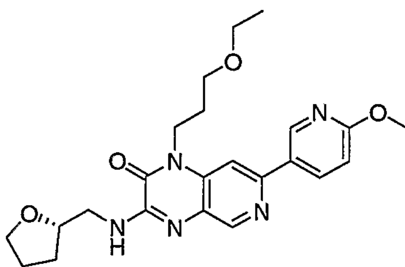
1-(3-ethoxypropyl)-7-(6-methoxypyridin-3-yl)-3-[(2S)-tetrahydrofuran-2-yl)methyl]amino]pyrido[3,4-b]pyrazin-2(1H)-one
