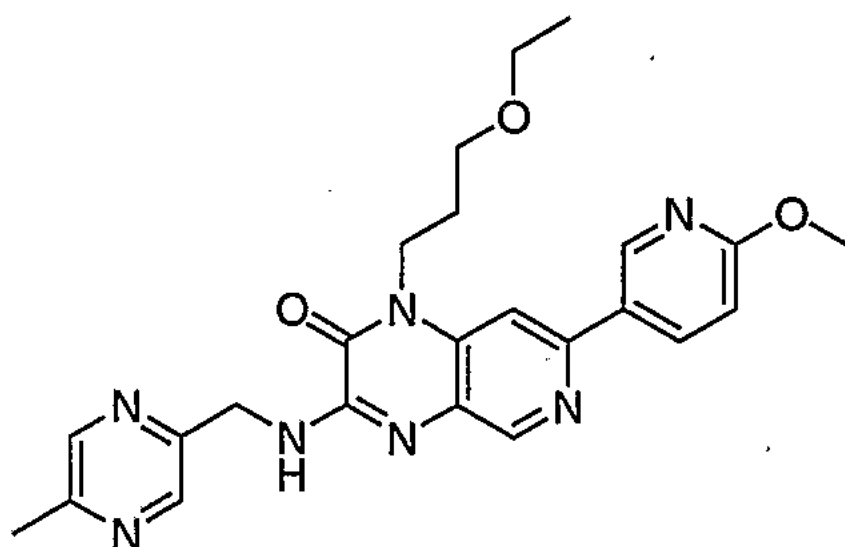
1-(3-ethoxypropyl)-7-(6-methoxypyridin-3-yl)-3-[[5-methylpyrazin-2-yl)methyl]amino]pyrido[3,4-b]pyrazin-2(1H)-one
