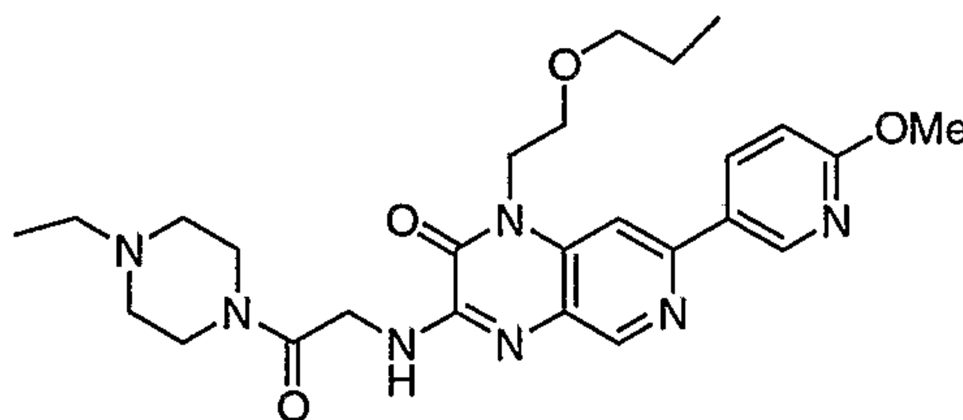
3-(2-(4-ethylpiperazin-1-yl)-2-oxoethylamino)-7-(6-methoxypyridin-3-yl)-1-(2-propoxyethyl)pyrido[3,4-b]pyrazin-2(1H)-one
