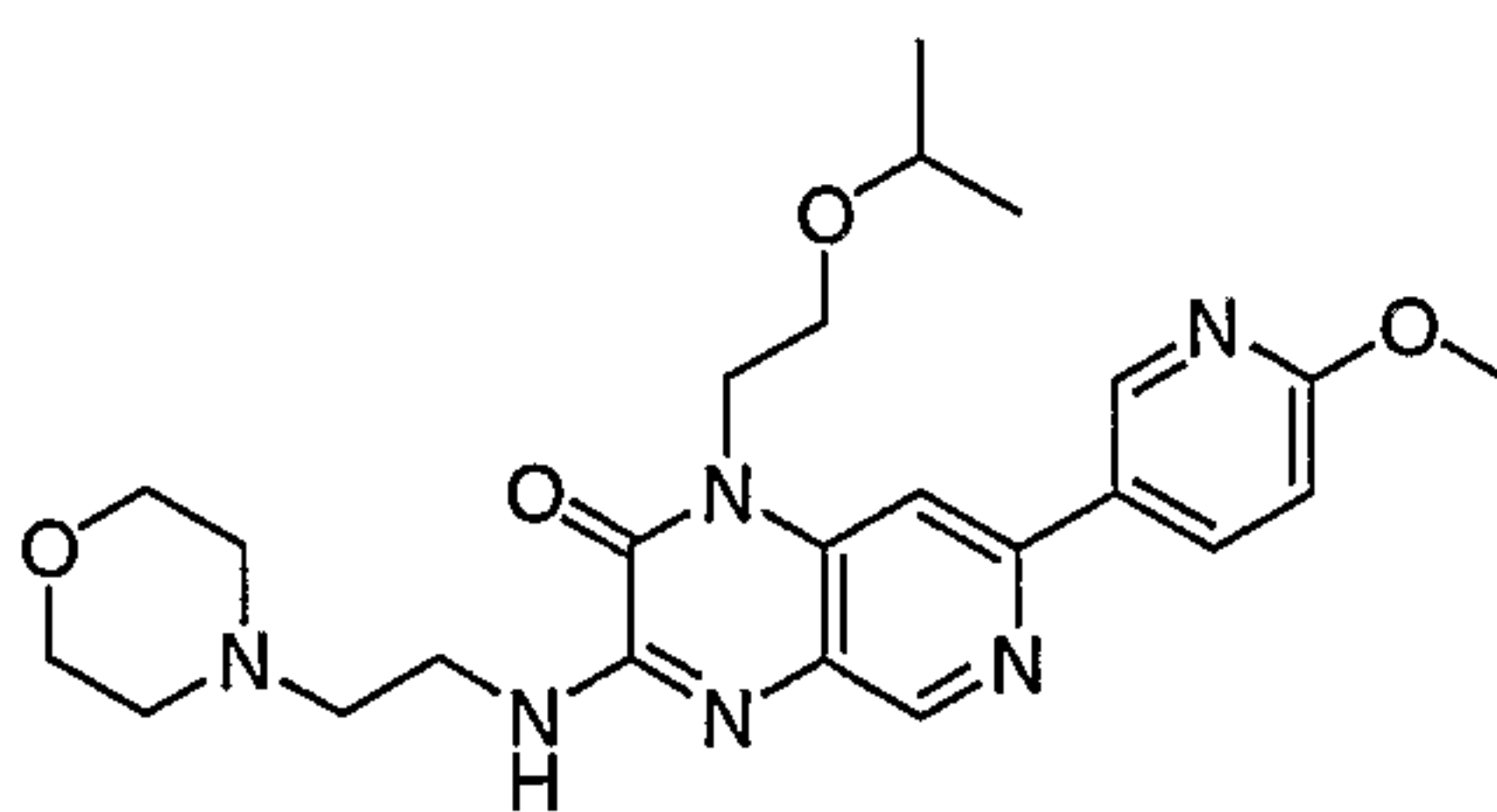
3-(2-morpholinoethylamino)-1-(2-isopropoxyethyl)-7-(6-methoxypyridin-3-yl)pyrido[3,4-b]pyrazin-2(1H)-one
