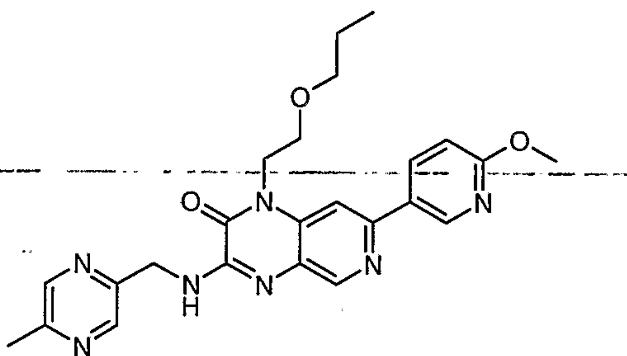
7-(6-methoxypyridin-3-yl)-3-[[5-methylpyrazin-2-yl)methyl]amino]-1-(2-propoxyethyl)pyrido[3,4-b]pyrazin-2(1H)-one.
