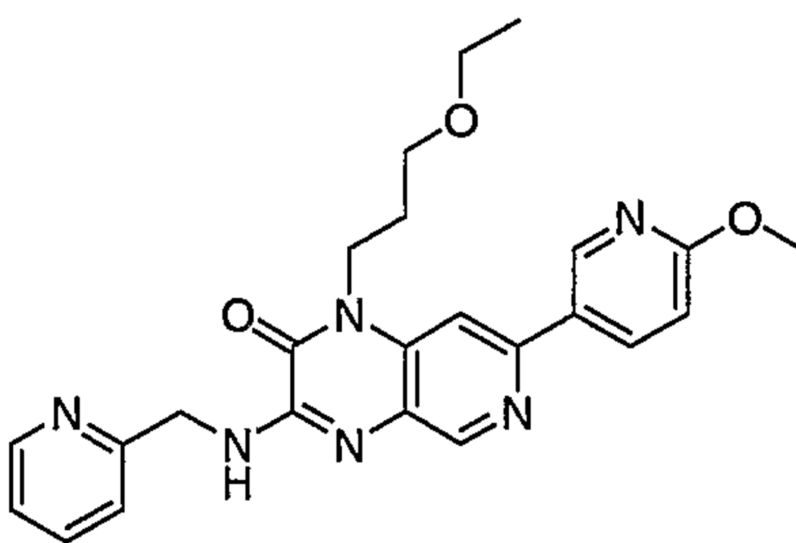
1-(3-ethoxypropyl)-7-(6-methoxypyridin-3-yl)-3-[(pyridin-2-ylmethyl)amino]pyrido[3,4-b]pyrazin-2(1H)-one
