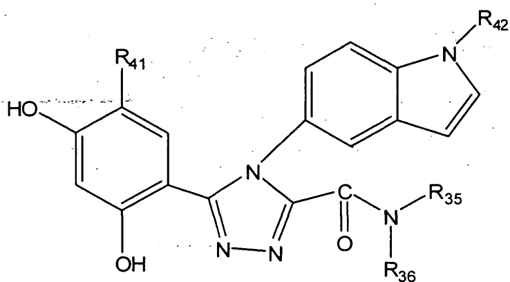
(XIV)
