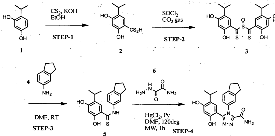
Scheme VI
