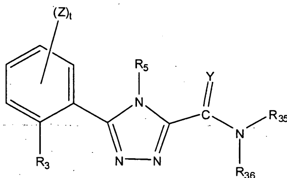
(VIII)
