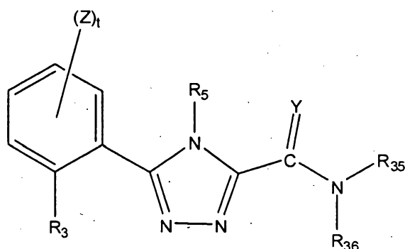
(VIII)
