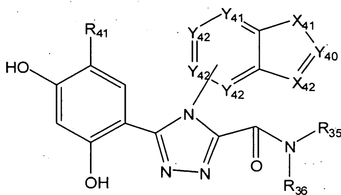
(XI)
