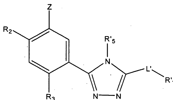
(III)
