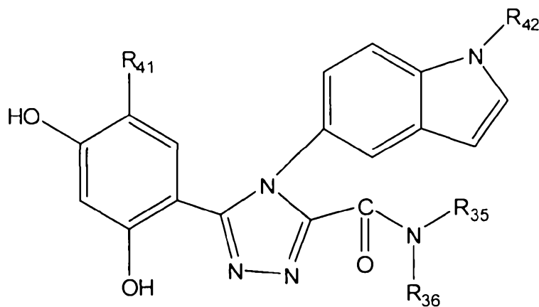
(XIV)
