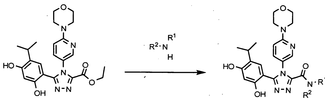
Scheme VI
