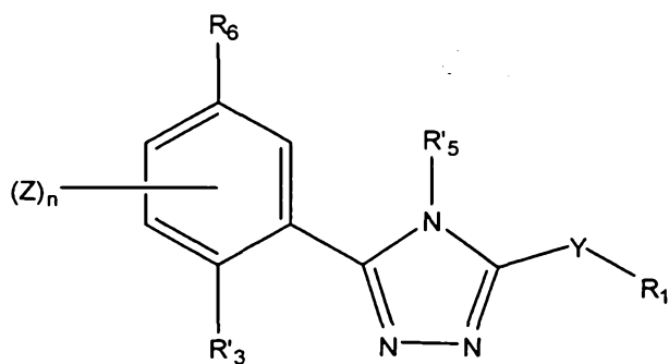
(XV)
