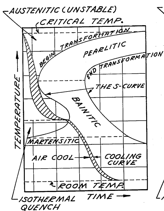
MAR-QUENCHING FIG. 8
