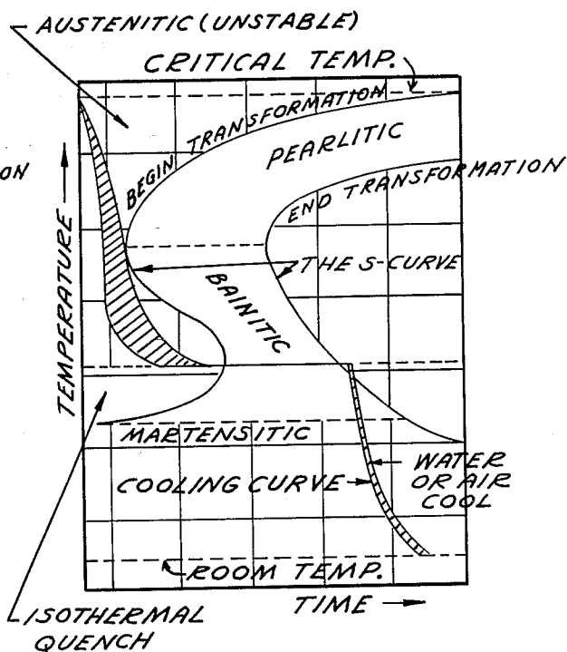
AUS-TEMPERING FIG. 7
