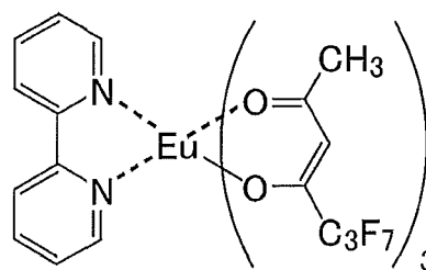
[Eu(FPD) 3 ]bpy
