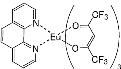
Eu(HFA) 3 phen
