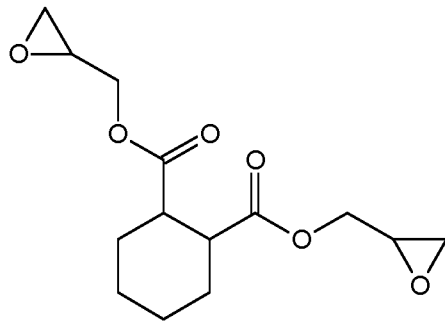
Hexahydrophthalsäurediglycidylether
