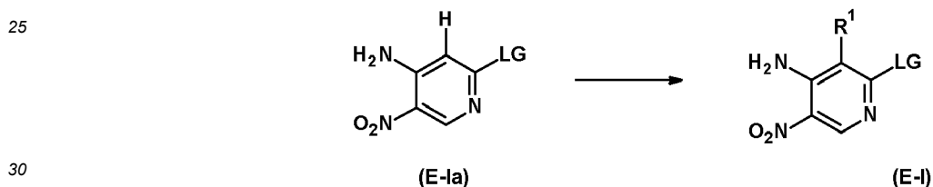
Schema 2.
