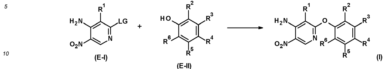
Schema 1.
