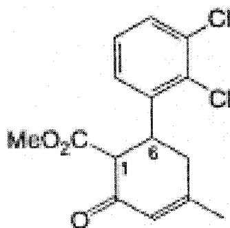
Substance 25 (1,6 trans)
