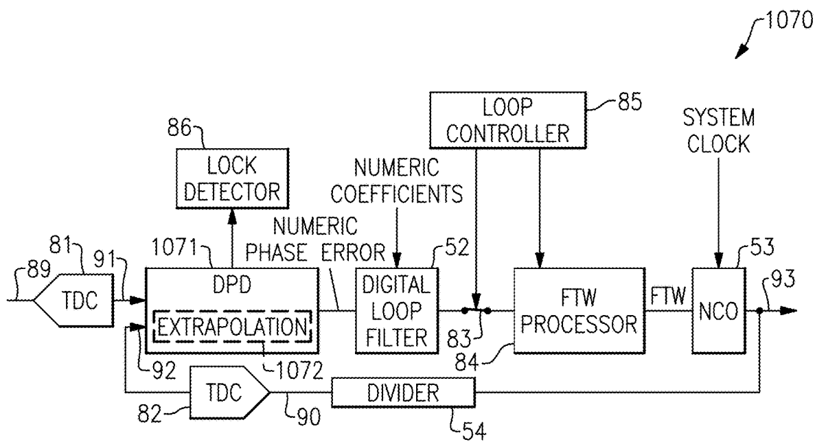
FIG.32
