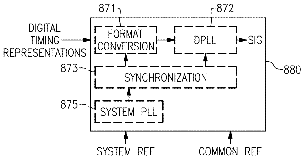
FIG.27B
