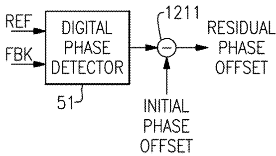
FIG.35A
