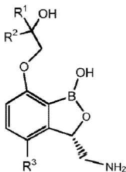
Formule IIIa
