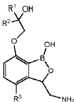
Formule III
