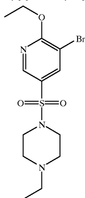
3-Bromo-2-ethoxy-5-(4-ethylpiperazin-1-ylsulphonyl)pyridine
