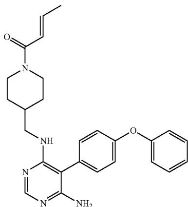
(E)-1-(4-(((6-amino-5-(4-phenoxyphenyl)pyrimidin-4-yl)amino)methyl)piperidin-1-yl)but-2-en-1-one (A13)
