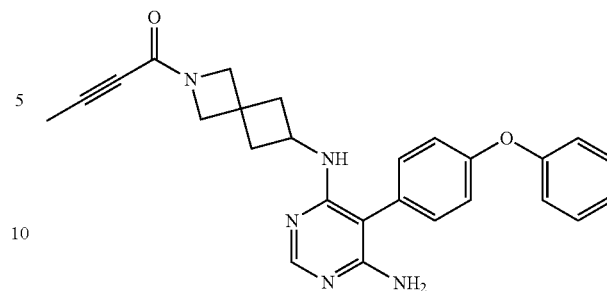
1-(6-((6-amino-5-(4-phenoxyphenyl)pyrimidin-4-yl)amino)-2-azaspiro[3.3]heptan-2-yl)but-2-yn-1-one (A108)
