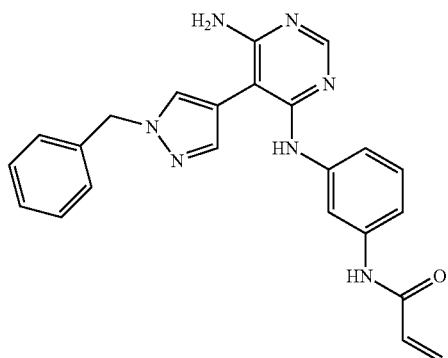
N-3-(((6-amino-5-(1-benzyl-1H-pyrazol-4-yl)pyrimidin-4-yl)amino)phenyl)acrylamide (A70)
