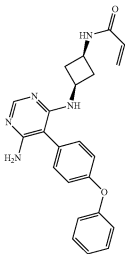
N-((1,3-cis-3-((6-amino-5-(4-phenoxyphenyl)pyrimidin-4-yl)amino)cyclobutyl)acrylamide (A118)
