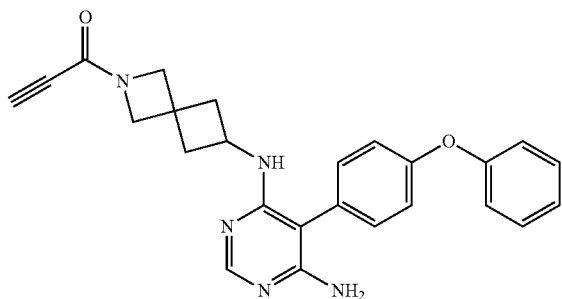
1-((6-amino-5-(4-phenoxyphenyl)pyrimidin-4-yl)amino)-2-azaspiro[3.3]heptan-2-yn-1-one
