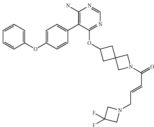
(E)-1-(6-(((6-amino-5-(4-phenoxyphenyl)pyrimidin-4-yl)oxy)-2-azaspiro[3.3]heptan-2-yl)-4-(3,3-difluoroazetidin-1-yl)but-2-en-1-one (A223)
