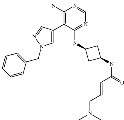
(E)-N-(1,3-cis-3-((6-amino-5-(1-benzyl-1H-pyrazol-4-yl)pyrimidin-4-yl)amino)cyclobutyl)-4-(dimethylamino)but-2-enamide (A230)
