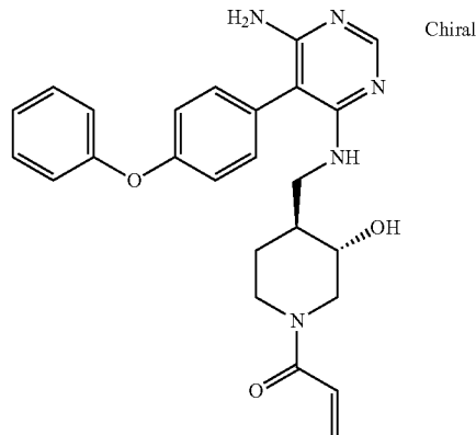
1-((3S,4S)-4-(((6-amino-5-(4-phenoxyphenyl)pyrimidin-4-yl)amino)methyl)-3-hydroxypiperidin-1-yl)prop-2-en-1-one
