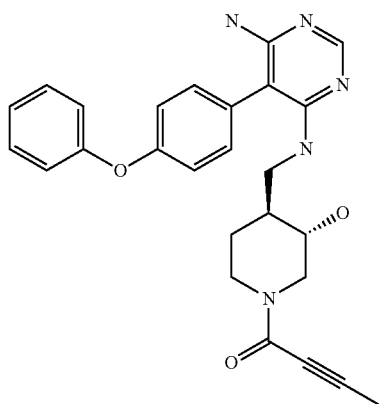
1-((3S,4S)-4-(((6-amino-5-(4-phenoxyphenyl)pyrimidin-4-yl)amino)methyl)-3-hydroxypiperidin-1-yl)but-2-yn-1-one (A215)
