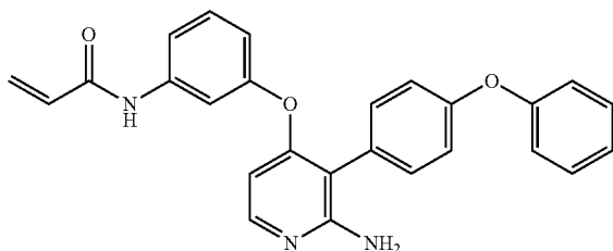
N-(3-((2-amino-3-(4-phenoxyphenyl)pyridin-4-yl)oxy)phenyl)acrylamide (A244)
