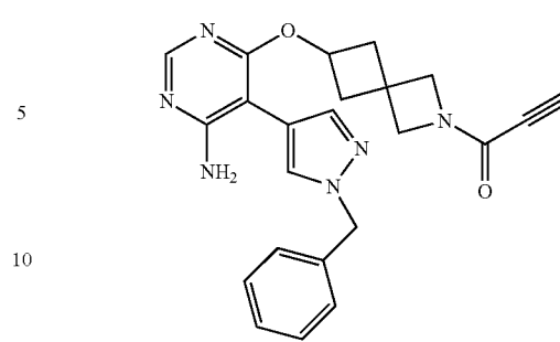
1-(6-(((6-amino-5-(1-benzyl-1H-pyrazol-4-yl)pyrimidin-4-yl)oxy)-2-azaspiro[3.3]heptan-2-yl)prop-2-yn-1-one (A112)
