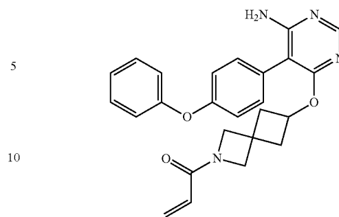
1-(6-((6-amino-5-(4-phenoxyphenyl)pyrimidin-4-yl)oxy)-2-azaspiro[3.3]heptan-2-yl) prop-2-en-1-one (A120)
