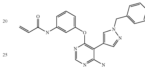
N-3-(((6-amino-5-(1-benzyl-1H-pyrazol-4-yl)pyrimidin-4-yl)oxy)phenyl)acrylamide (A172)
