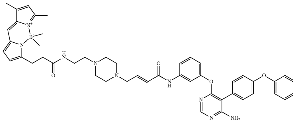
(E)-7-(3-((2-(4-(4-(((6-amino-5-(4-phenoxyphenyl)pyrimidin-4-yl)oxy)phenyl)amino)-4-oxobut-2-en-1-yl)piperazin-1-yl)ethyl)amino)-3-oxopropyl)-5,5-difluoro-1,3-dimethyl-5H-dipyrrolo[1,2-c:2',1'-f][1,3,2]diazaborinin-4-ium-5-uide (A35)
