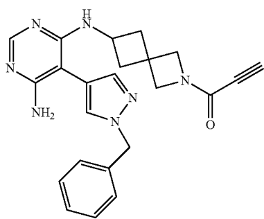
1-((6-(((6-amino-5-(1-benzyl-1H-pyrazol-4-yl)pyrimidin-4-yl)amino)-2-azaspiro[3.3]heptan-2-yl)prop-2-yn-1-one (A111)
