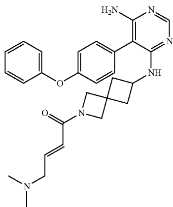
(E)-1-(6-(((6-amino-5-(4-phenoxyphenyl)pyrimidin-4-yl)amino)-2-azaspiro[3.3]heptan-2-yl)-4-(dimethylamino)but-2-en-1-one (A127)
