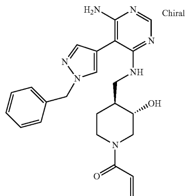
1-((3S,4S)-4-(((6-amino-5-(1-benzyl-1H-pyrazol-4-yl)pyrimidin-4-yl)amino)methyl)-3-hydroxypiperidin-1-yl)prop-2-en-1-one (A109)
