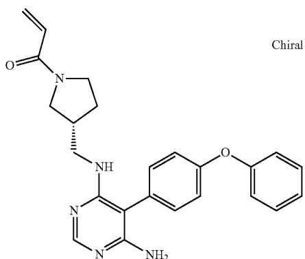
(R)-1-(3-(((6-amino-5-(4-phenoxyphenyl)pyrimidin-4-yl)amino)methyl)pyrrolidin-1-yl)prop-2-en-1-one (A4)
