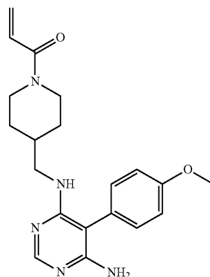
1-(4-(((6-amino-5-(4-methoxyphenyl)pyrimidin-4-yl)amino)methyl)piperidin-1-yl)prop-2-en-1-one (A85)
