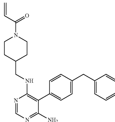
1-(4-(((6-amino-5-(4-benzylphenyl)pyrimidin-4-yl)amino)methyl)piperidin-1-yl)prop-2-en-1-one (A41)
