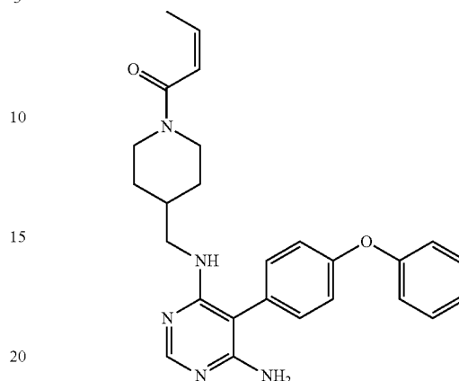
(Z)-1-(4-(((6-amino-5-(4-phenoxyphenyl)pyrimidin-4-yl)amino)methyl)piperidin-1-yl)but-2-en-1-one (A15)
