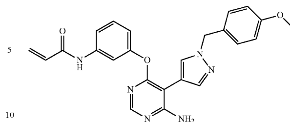
N-3-(((6-amino-5-(1-(4-methoxybenzyl)-1H-pyrazol-4-yl)pyrimidin-4-yl)oxy)phenyl)acrylamide (A72)
