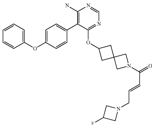
(E)-1-(6-(((6-amino-5-(4-phenoxyphenyl)pyrimidin-4-yl)oxy)-2-azaspiro[3.3]heptan-2-yl)-4-(3-fluoroazetidin-1-yl)but-2-en-1-one (A222)
