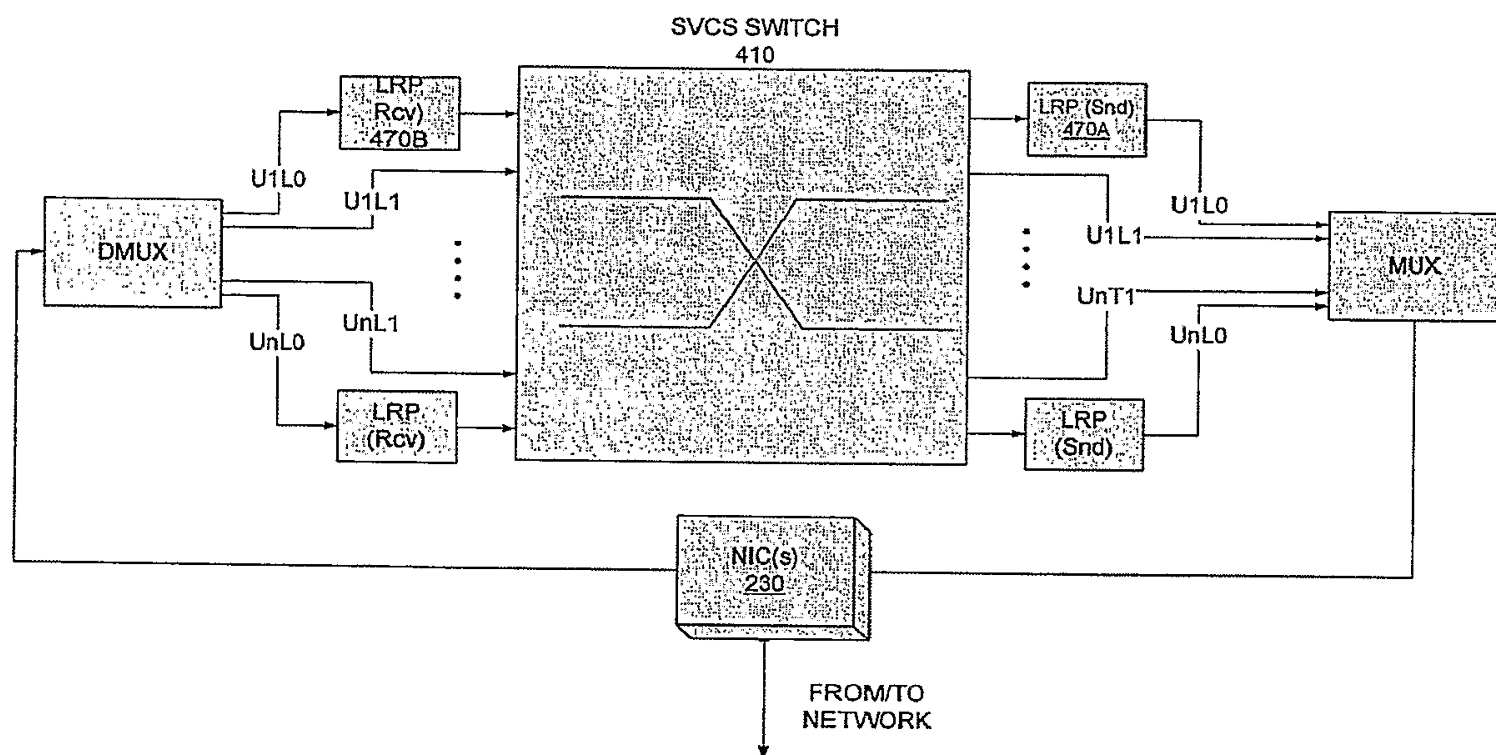
FIG. 4: SVCS
