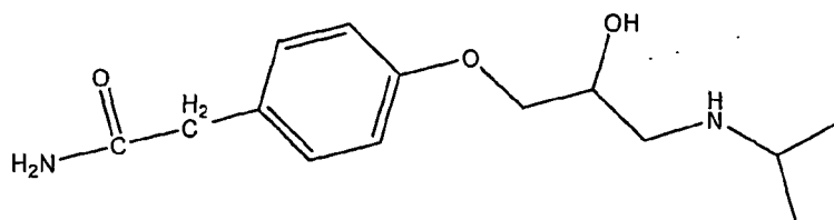
Atenolol
