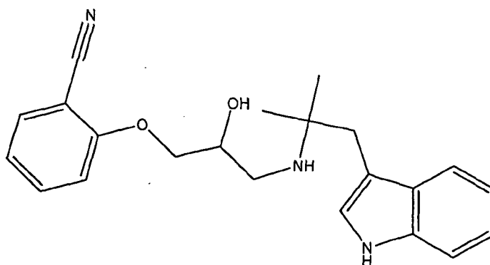
Bucindolol
