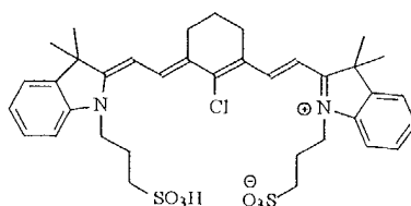
IR Dye A
