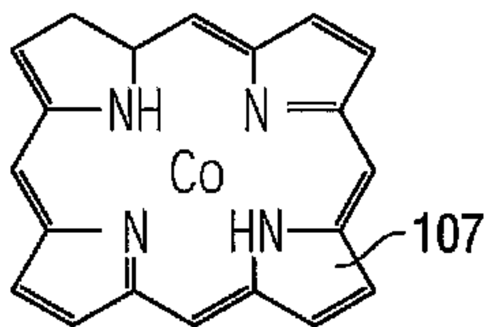
A Porphyrin
